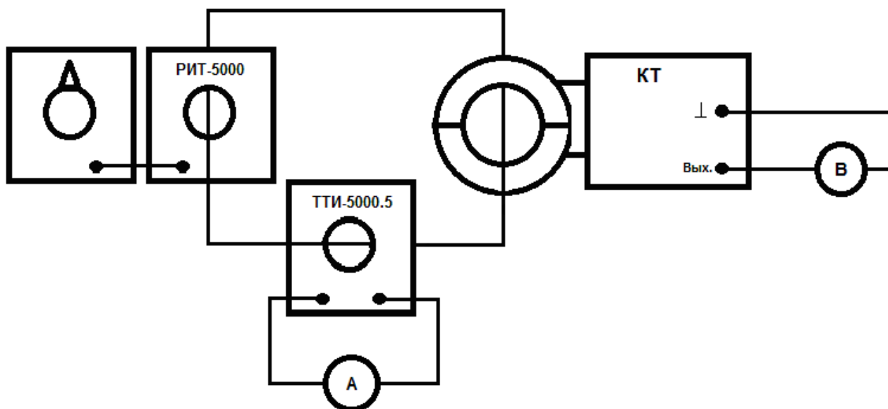
Рисунок 10 – Схема измерений при определении погрешности преобразования силы переменного тока для клещей токоизмерительных КТ-***-П-Д54
