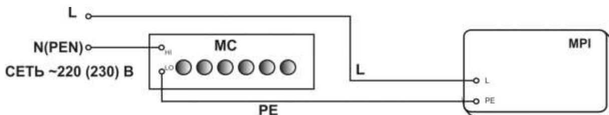
Рисунок 12 – Структурная схема определения абсолютной погрешности измерения действующего значения напряжения прикосновения,
