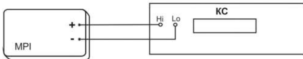
Рисунок 20 – Структурная схема определения абсолютной погрешности измерения сопротивления электроизоляции,
