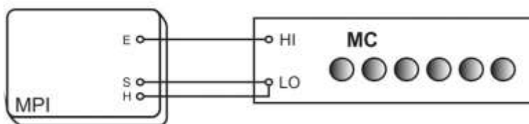
Рисунок 15 - Структурная схема определения абсолютной погрешности измерения сопротивления заземляющего устройства без использования клещей трехполюсным методом, где MPI – поверяемый измеритель,
