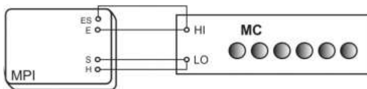
Рисунок 16 - Структурная схема определения абсолютной погрешности измерения сопротивления заземляющего устройства без использования клещей 4х полюсным методом,
