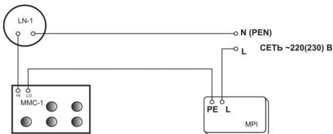
Рисунок 8 - Структурная схема определения абсолютной погрешности измерения полного сопротивления цепи “фаза-защитный проводник”,
