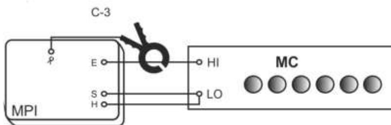
Рисунок 17 - Структурная схема определения абсолютной погрешности измерения электрического сопротивления заземляющего устройства с использованием клещей, где MPI – поверяемый измеритель, MC – магазин электрического сопротивления MC-6-01/03, С-3 – клещи измерительные С-3.
