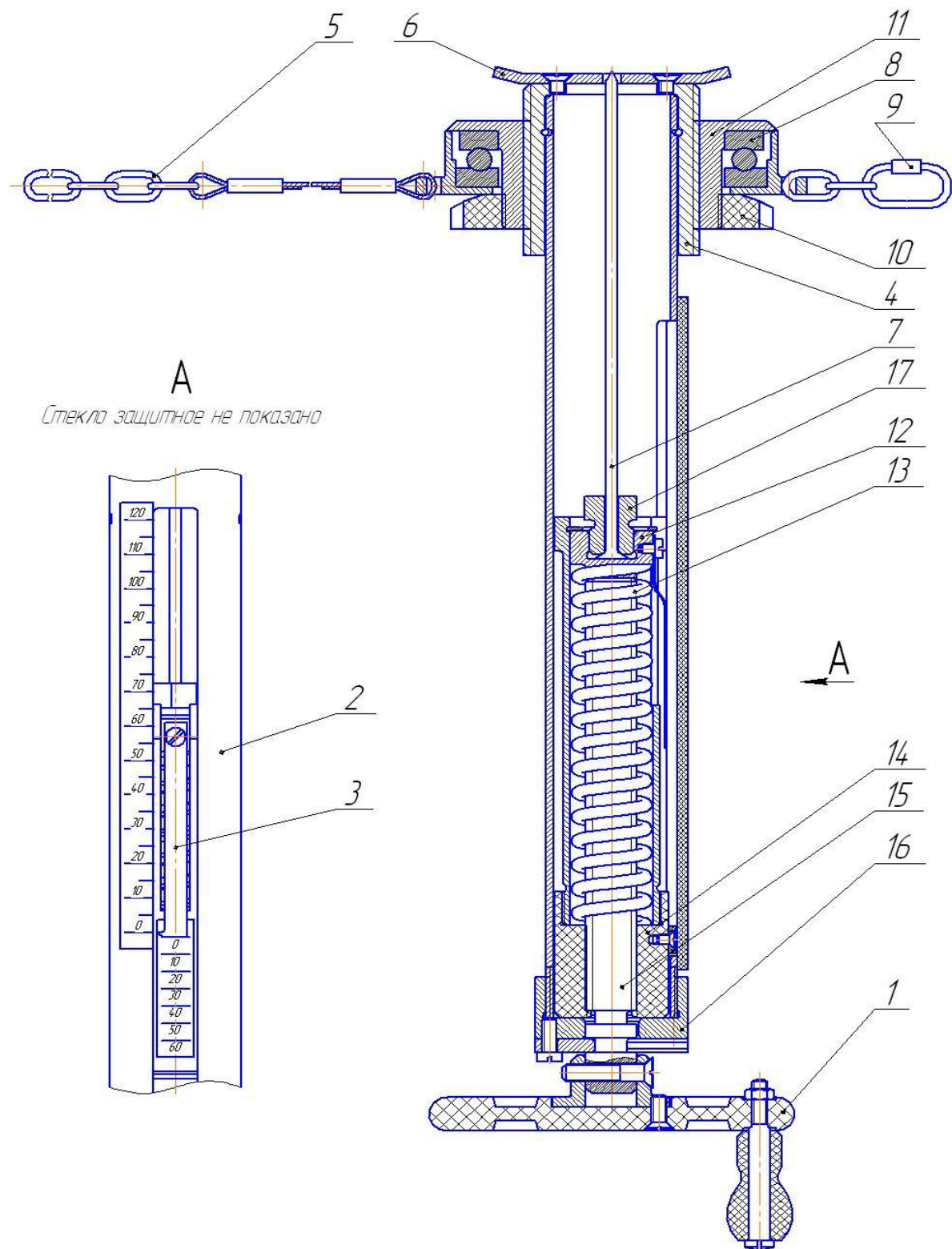
Рис.1. Общий вид устройства АКОД-М®
