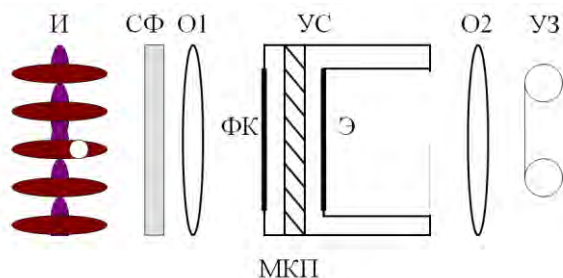
Рисунок 1 — Блок-схема ЭОД
