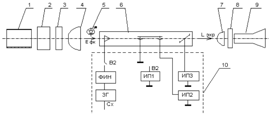
Рисунок 2 — Функциональная схема ЭОД «Филин-6»
