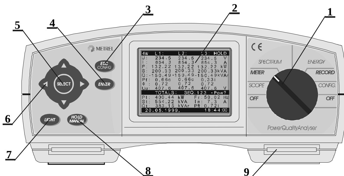
Рисунок 2 – Передняя панель
