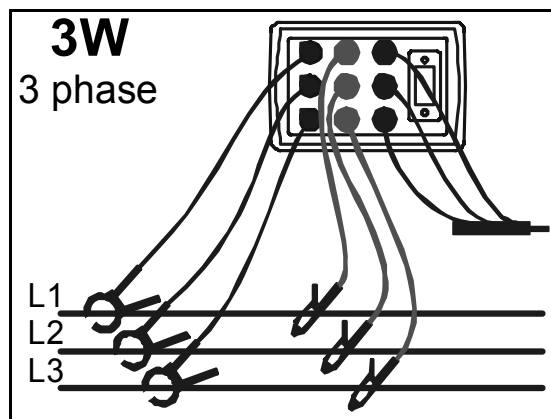
Рисунок 21 - 3фазная 3проводная система с тремя трансформаторами тока
