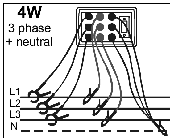
Рисунок 20 - 3фазная 4проводная система
