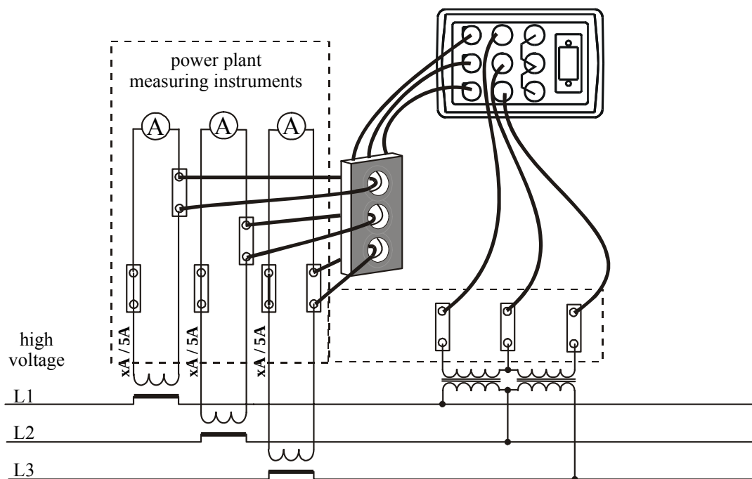
Рисунок 23 – Соединение к существующим трансформаторам тока в высоковольтной системе
