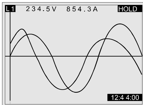
Рисунок 17 – Дисплей осциллографа без дополнительной информации
