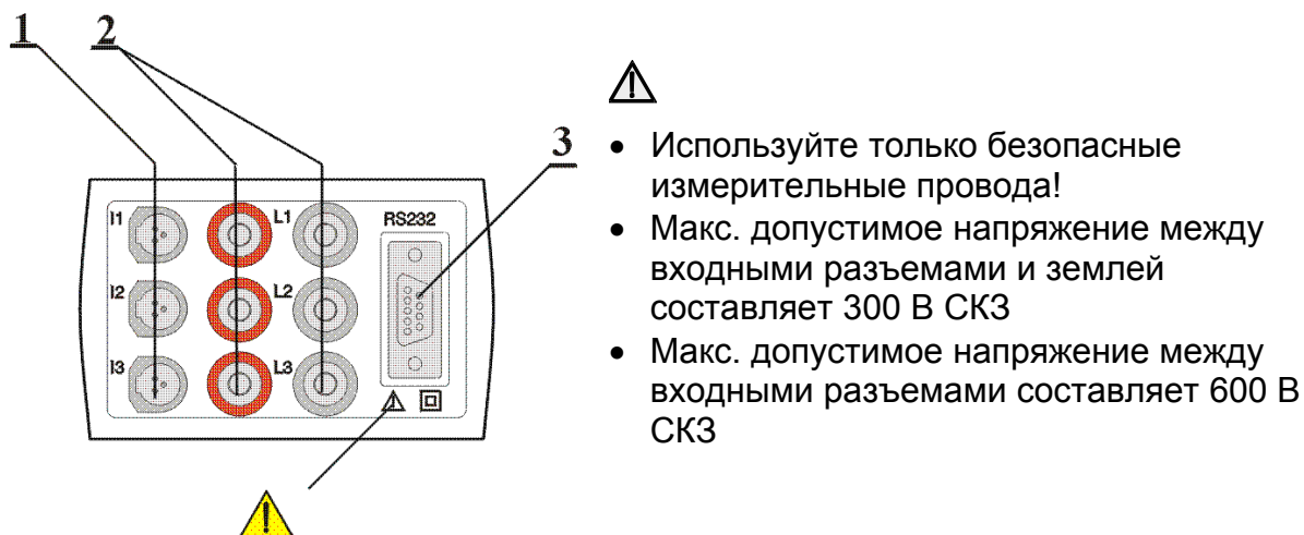
Рисунок 3 - Панель разъемов
