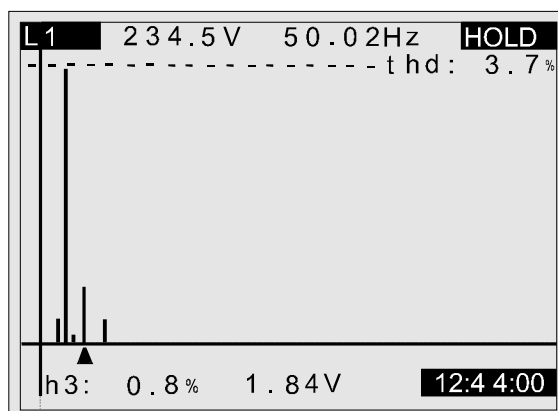
Рисунок 15 – Гармонический анализ
