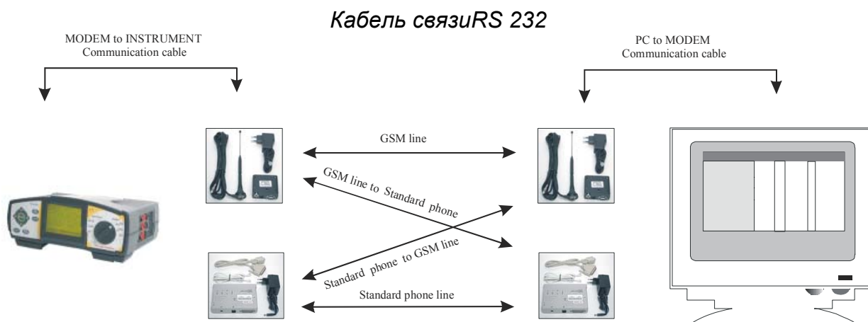
Подключение модема, прибора и ПК
