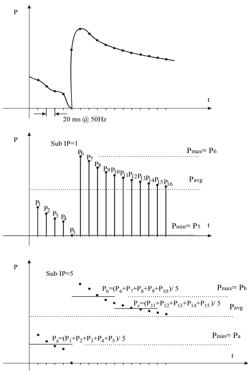
Рисунок 41 – Примеры вычисления максимума и минимума для разных подпериодов интегрирования мощности
