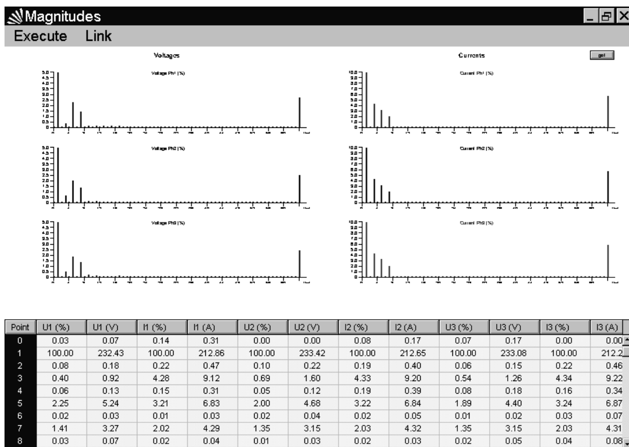
Рисунок 39 – Экран прямого гармонического анализа с табличным дисплеем
