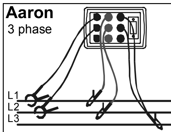
Рисунок 22 - 3фазная 3проводная система с двумя трансформаторами тока (соединение 2 ваттметров)
