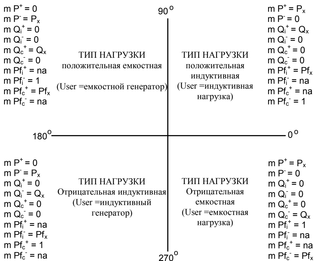
Рисунок 42 – Импорт/экспорт и индуктивная/емкостная фазная/полярная диаграмма
