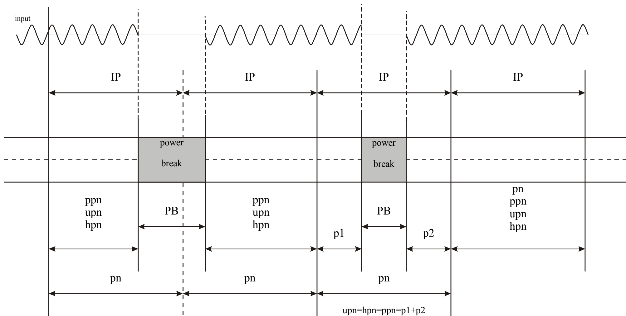
Рисунок 40 - Входные импульсы для вычисления в различных ситуациях обрыва питания
