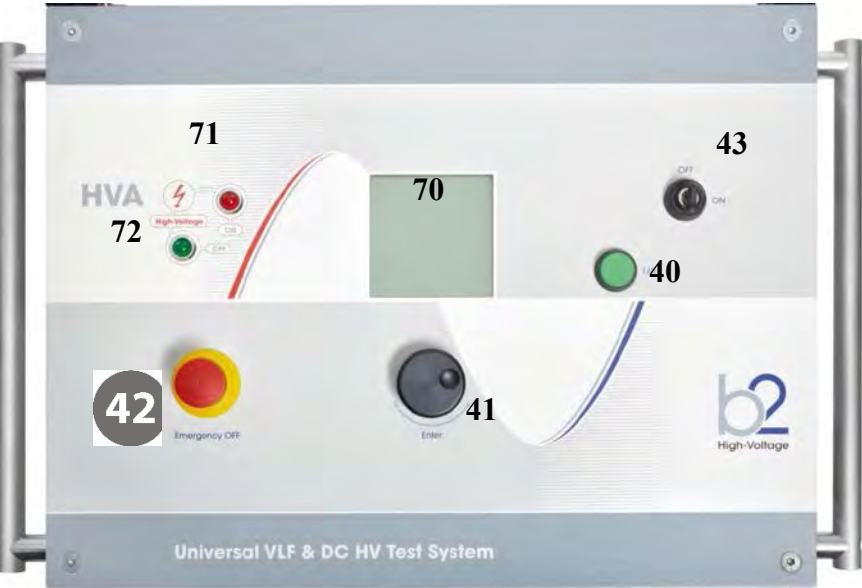
Рис 1: передняя панель
