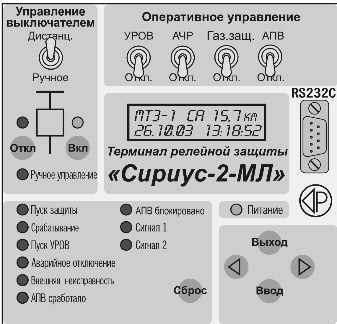
Рис.13. Расположение элементов управления и индикации на передней панели устройства «Сириус-2-МЛ»
