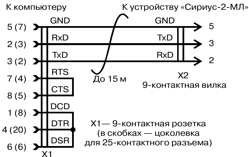
Рис.19. Схема соединительного кабеля между устройством «Сириус-2-МЛ» и компьютером при подключении только одного устройства
