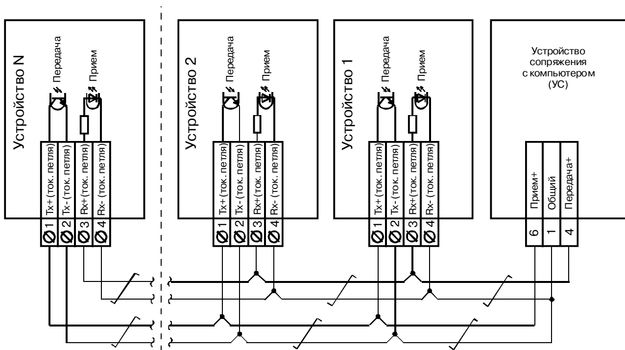
Рис. 20 Схема подключения устройств с интерфейсом «токовая петля» в локальную сеть. К каждому входу устройства сопряжения (всего четыре входа) может быть подключено до двадцати устройств защиты.
