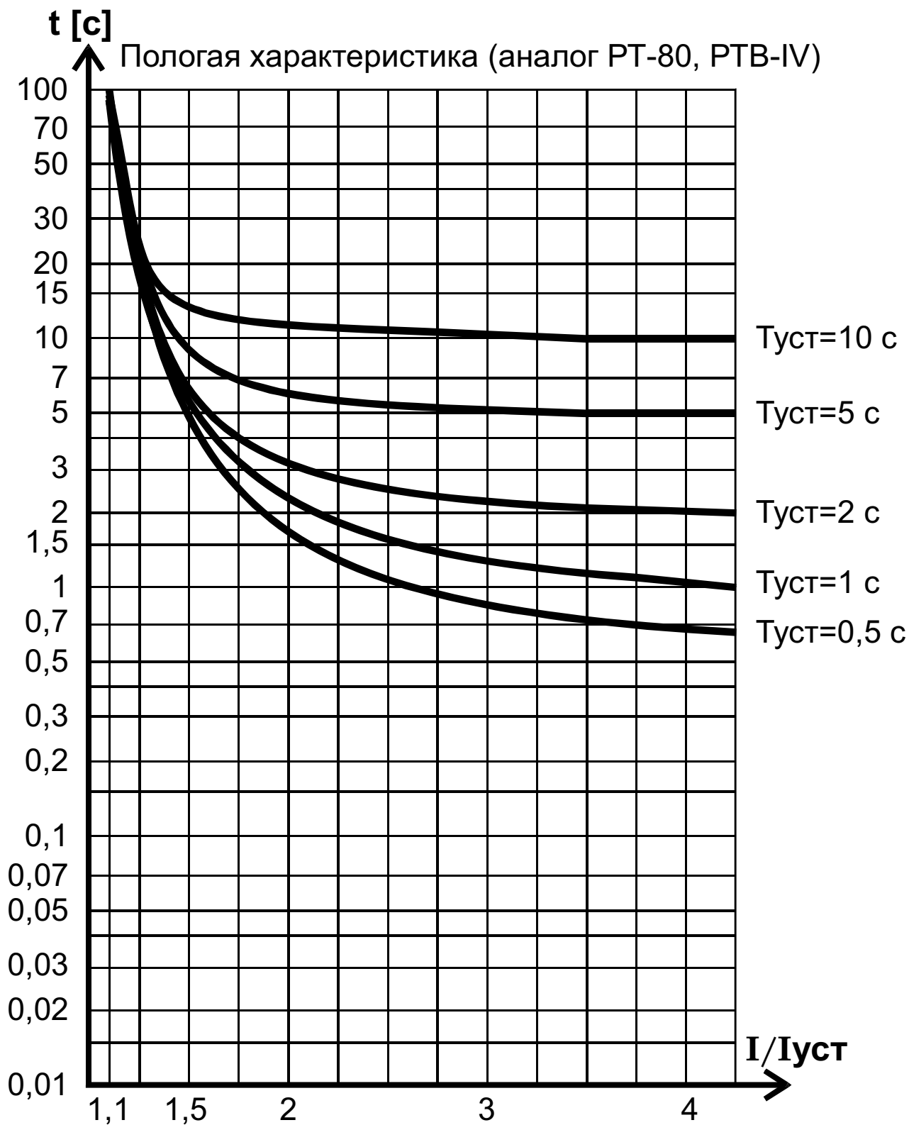
Рис.25. Пологая характеристика (аналог РТ-80, РТВ-IV)
