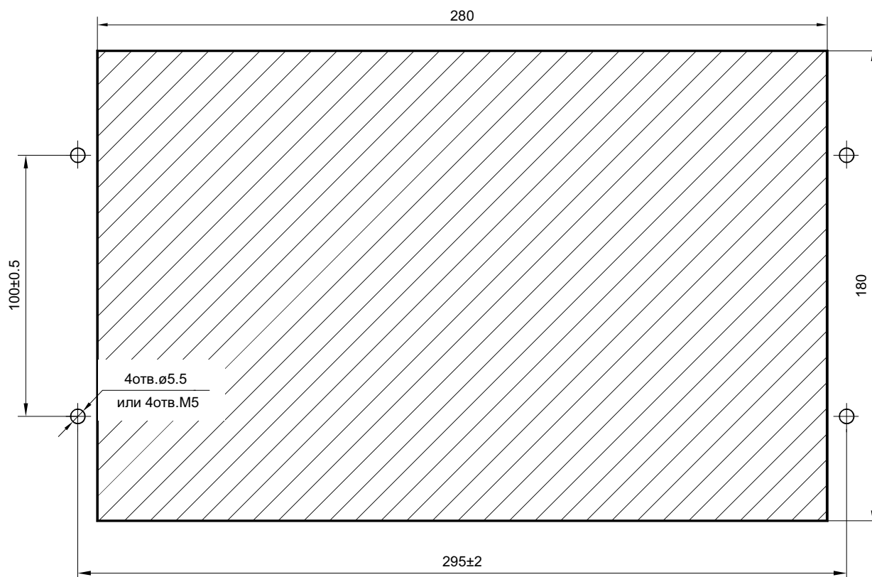
Рис. 15. Разметка панели под установку устройства «Сириус-2-МЛ»
