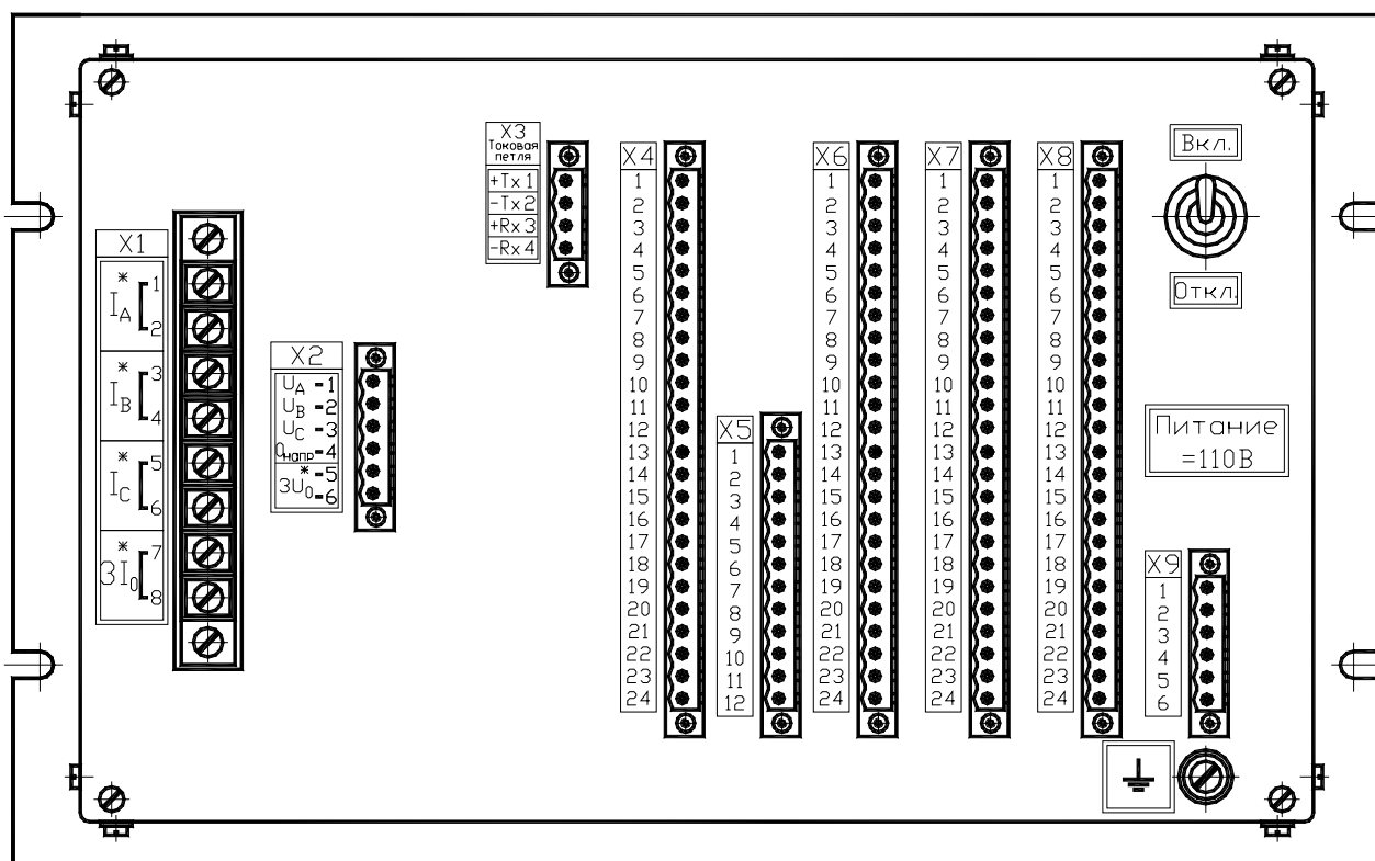
Рис. 14. Расположение элементов на задней панели устройства «Сириус-2-МЛ»
