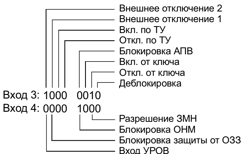
Рис.9. Соответствие входных дискретных сигналов в режиме «Контроль входов 3, 4». Активному состоянию соответствует «1», пассивному – «0».
