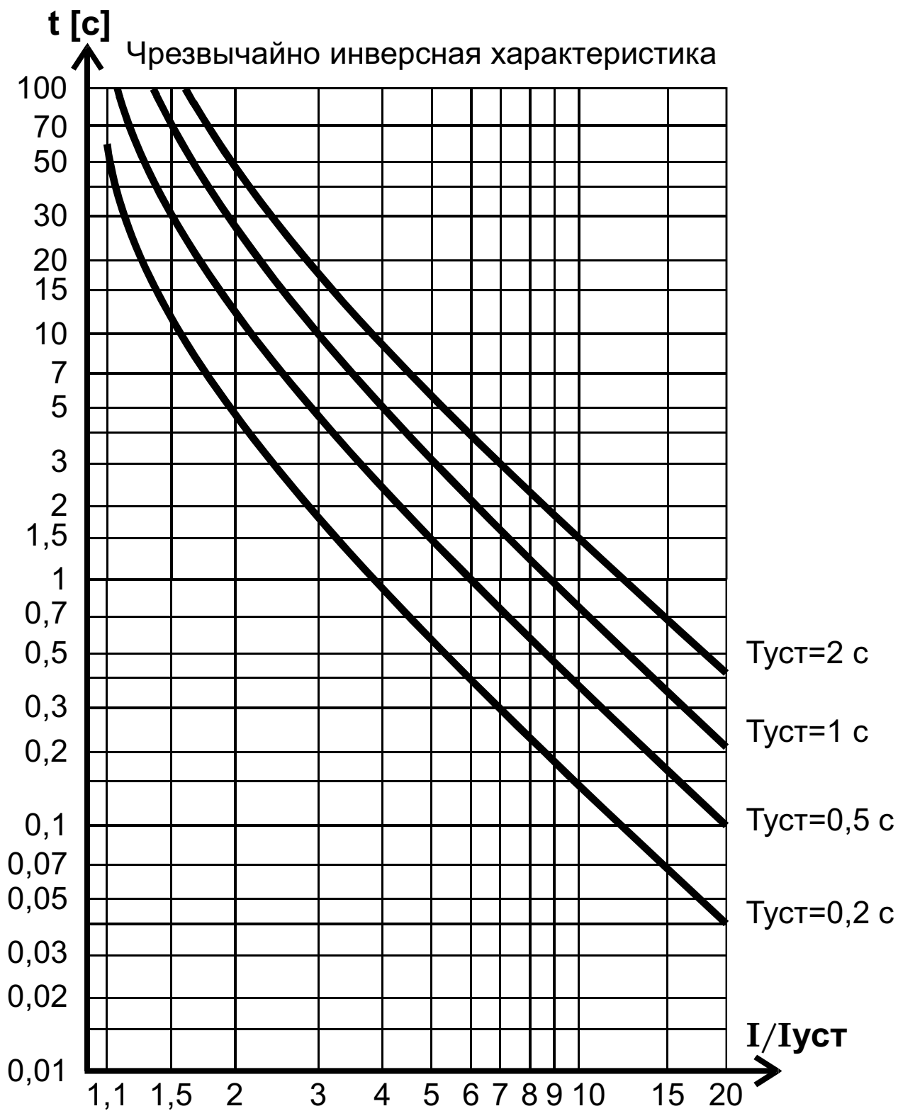
Рис.24. Чрезвычайно инверсная характеристика по МЭК 255-4
