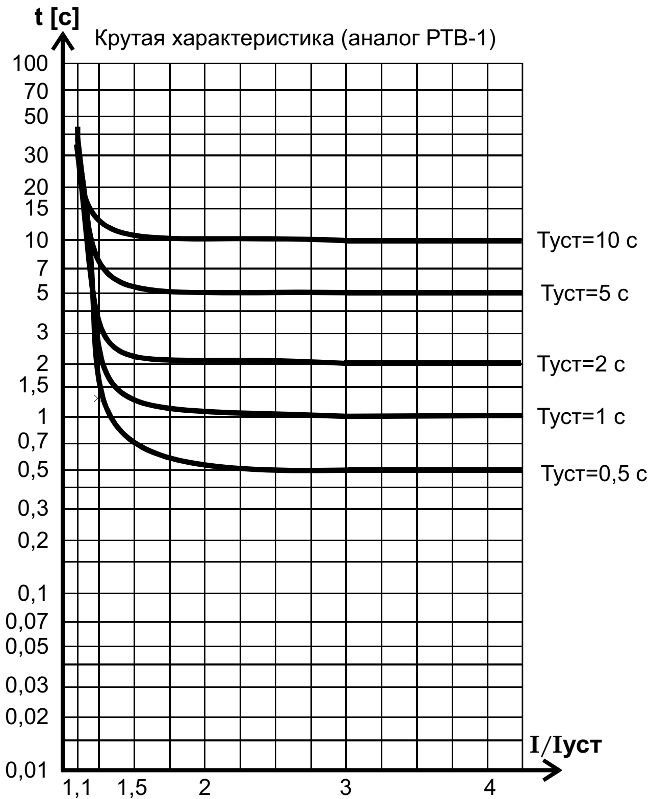
Рис.26. Крутая характеристика (аналог РТВ-1)
