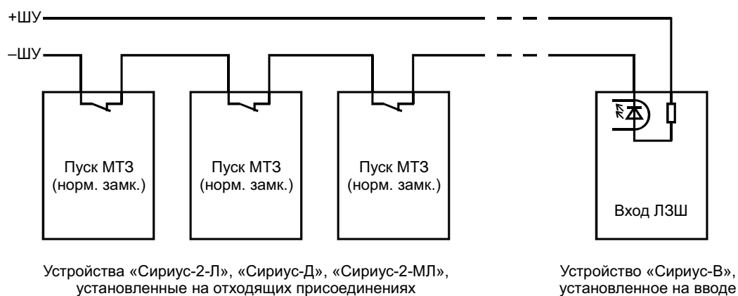
Рис.5б. Схема соединения нескольких устройств «Сириус-2-МЛ» между собой при организации логической защиты шин (последовательная схема)
