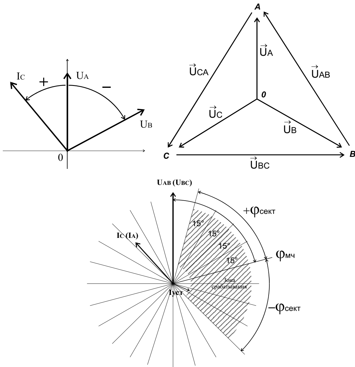
Рис.2. Поясняющие диаграммы определения направления мощности
