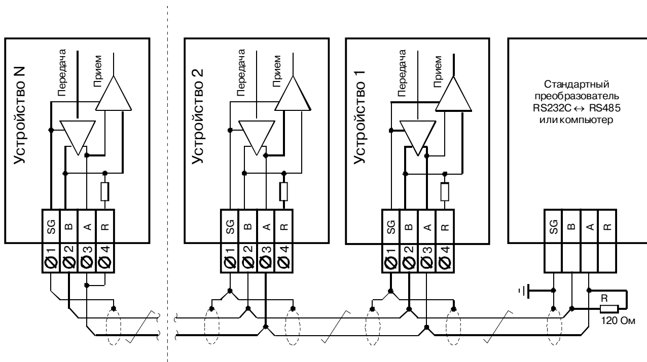
Рис. 21 Схема подключения устройств с интерфейсом RS485 в локальную сеть. Внешний резистор R устанавливается при отсутствии встроенного резистора.
