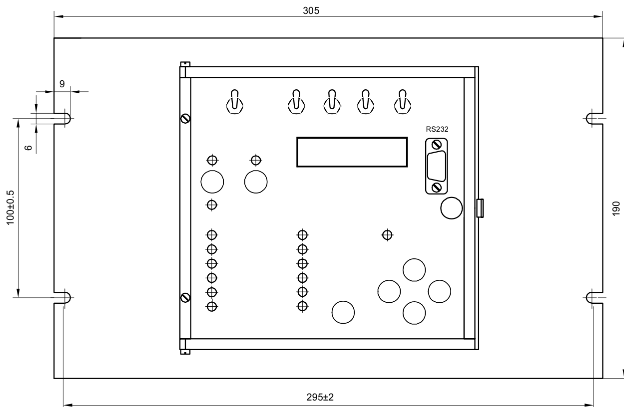
Рис.11. Устройство «Сириус-2-МЛ». Вид спереди.
