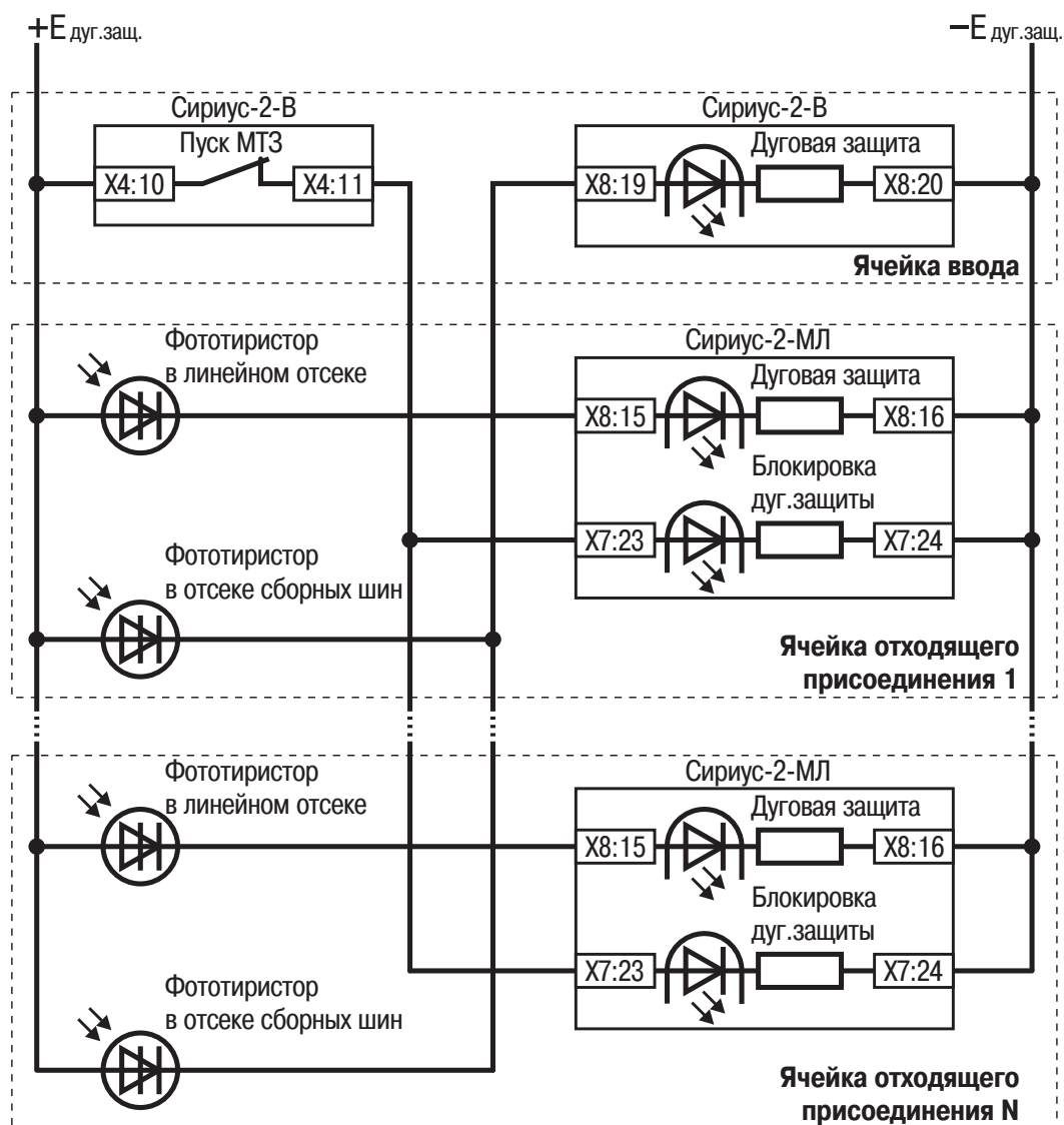
Рис.6. Упрощенная схема организации дуговой защиты с использованием контроля по току от защиты вводного выключателя
