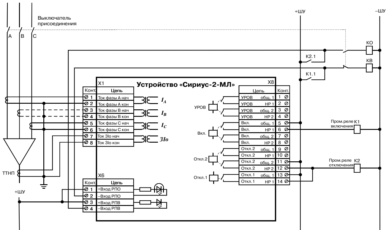
Рис.17. Фрагмент схемы подключения внешних цепей к устройству «Сириус-2-МЛ» при управлении выключателем через промежуточные реле
