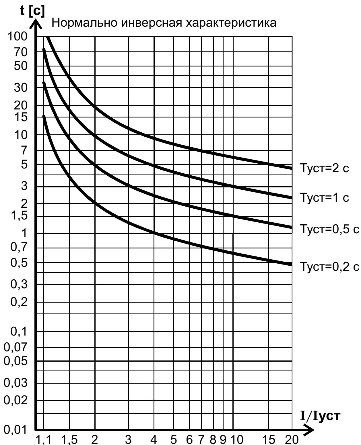
Рис.22. Нормально инверсная характеристика по МЭК 255-4
