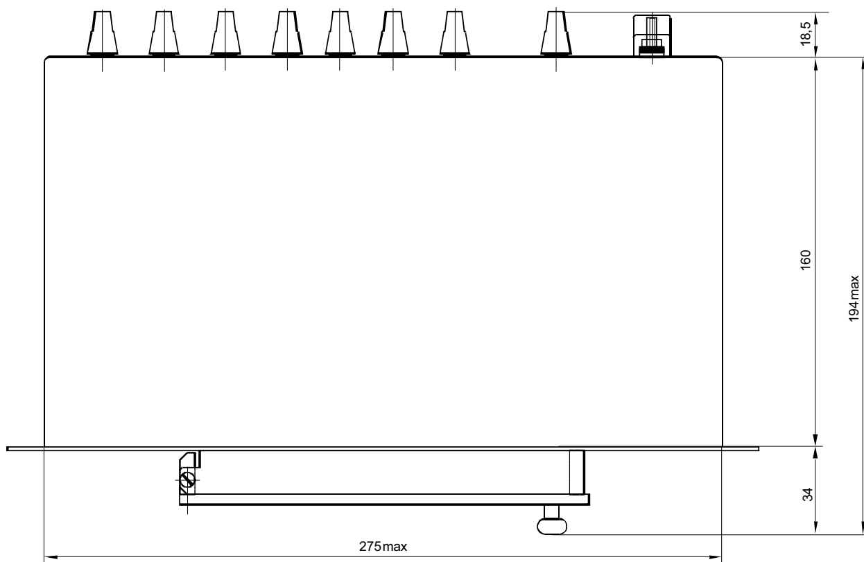
Рис.12. Устройство «Сириус-2-МЛ». Вид сверху.
