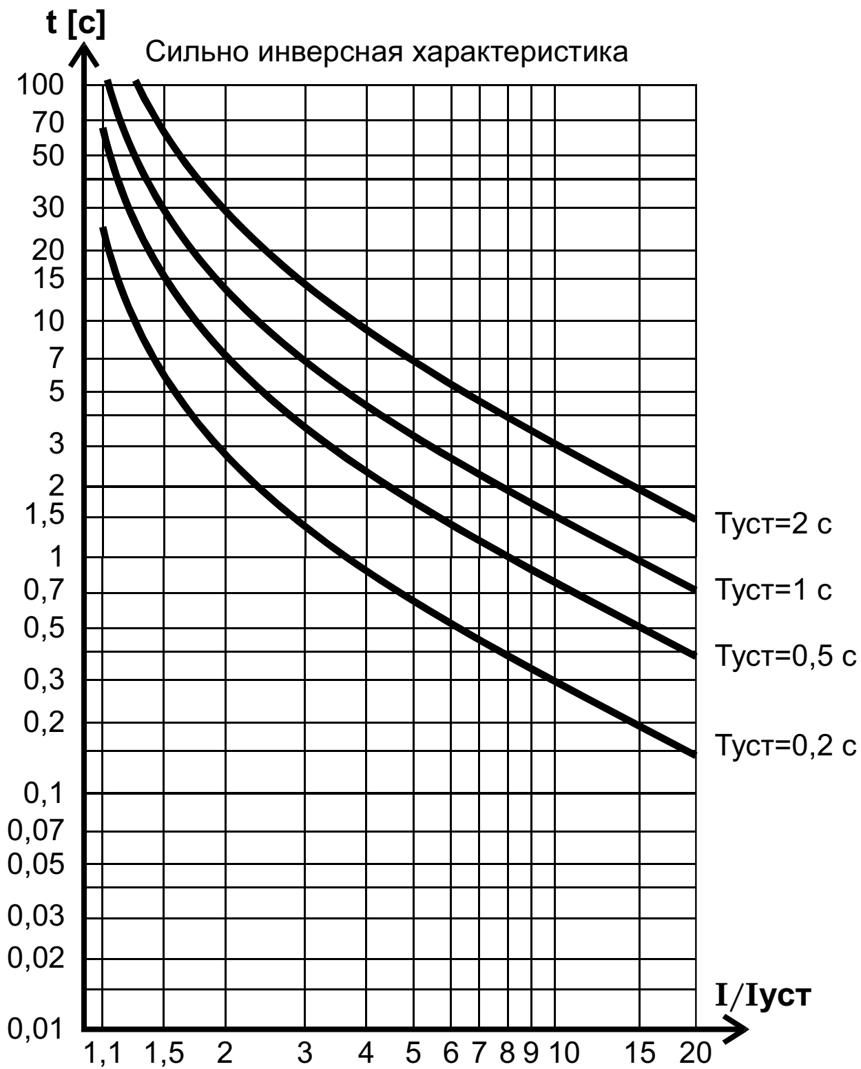
Рис.23. Сильно инверсная характеристика по МЭК 255-4
