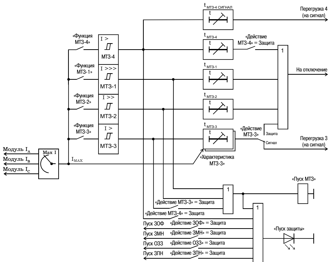
Рис.1. Фрагмент функциональной логической схемы построения МТЗ
