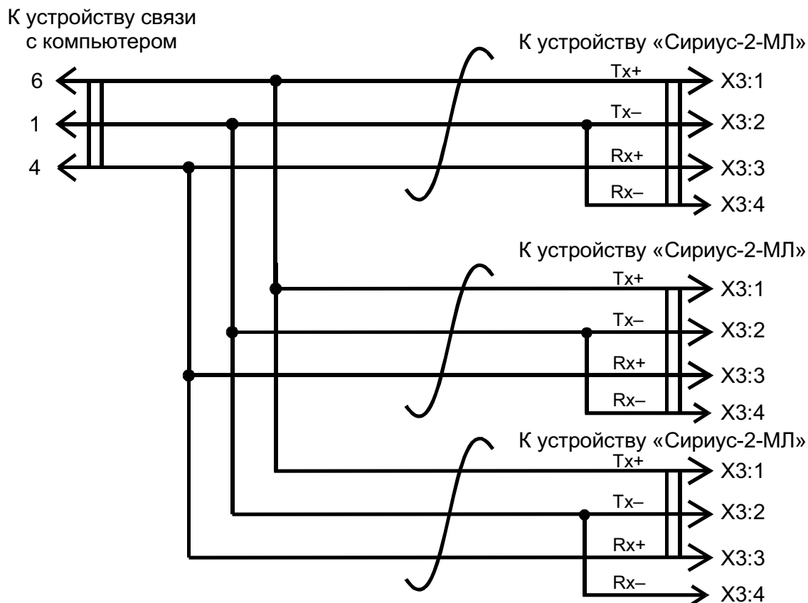
Рис.18. Схема соединительного кабеля между устройствами «Сириус-2-МЛ» и устройством сопряжения УС при использовании линии связи с компьютером
