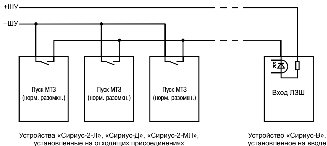
Рис.5а. Схема соединения нескольких устройств «Сириус-2-МЛ» между собой при организации логической защиты шин (параллельная схема)
