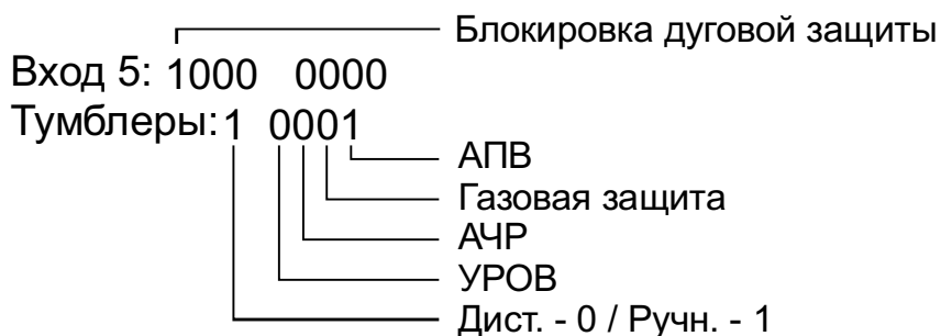
Рис. 10. Соответствие положения тумблеров оперативного управления, расположенных на передней панели устройства, в режиме «Контроль входов 5, контроль тумблеров». Включенному состоянию соответствует «1», отключенному – «0».
