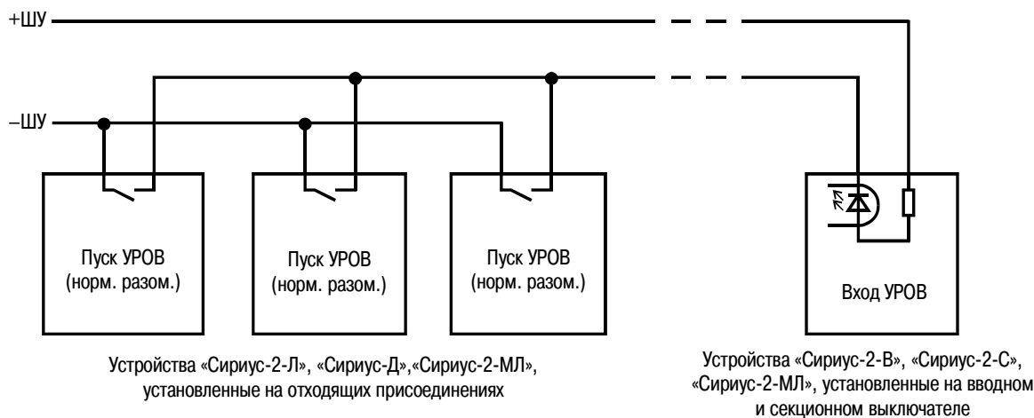
Рис.4. Схема организации УРОВ на подстанции
