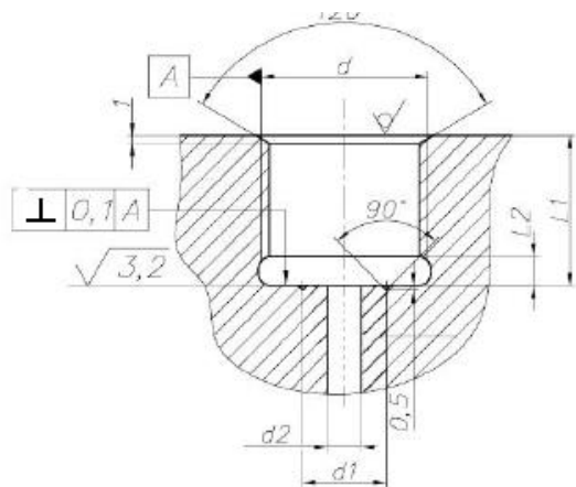
Рисунок Г.1 — Монтажное гнездо для преобразователей
