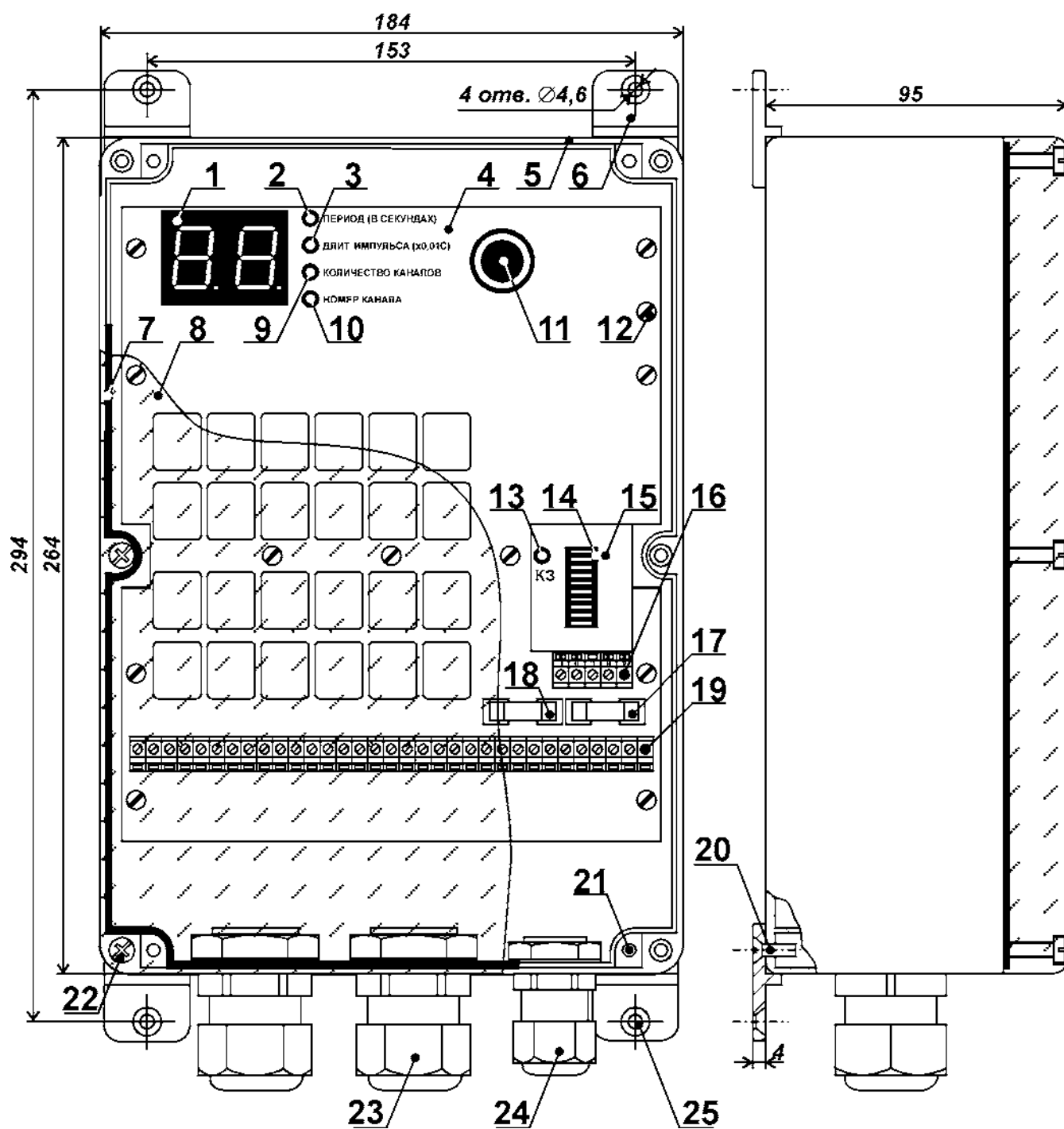
Рис. 1. Конструкция блока А-02-1.
