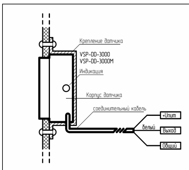
Рисунок 1. Датчик VSP-DD-3000(M)
