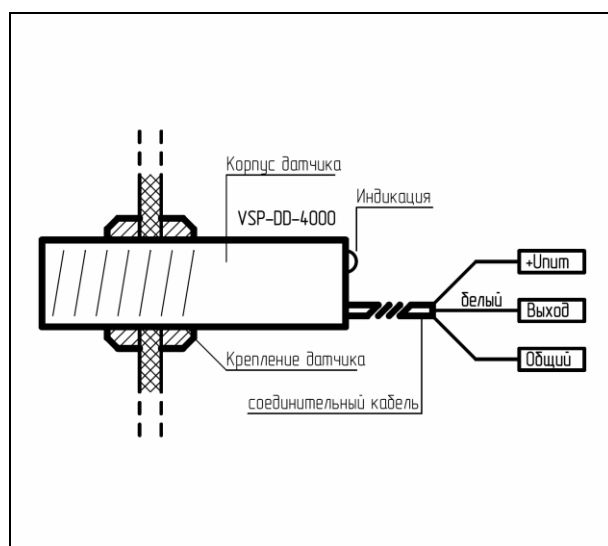
Рисунок 2. Датчик VSP-DD-4000
