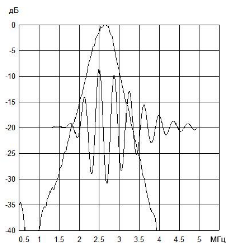
Форма и спектр эхо-сигнала для преобразователя П112-2,5-12-B-002
