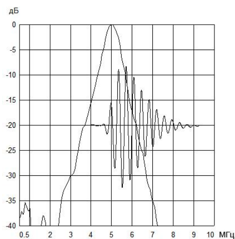
Форма и спектр эхо-сигнала для преобразователя П112-5-3x4-B-002
