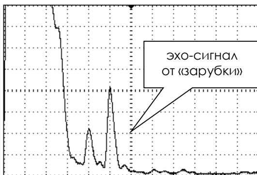
Эхо-сигнал от углового отражателя размером 1,5 x 0,8 мм на глубине 4 мм для преобразователя П121-10-75-400
