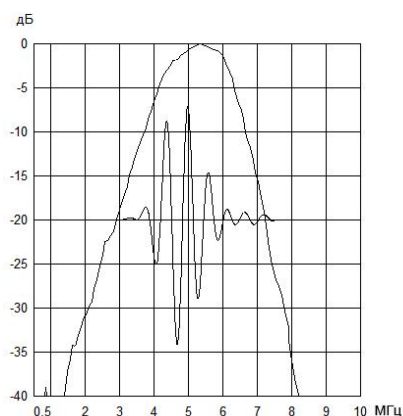
Эхо-сигнал от плоскости для преобразователя П112-5-10/2-T-01
