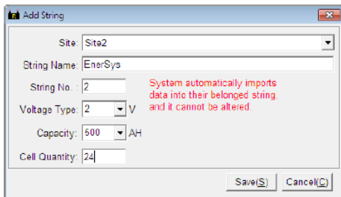
Рисунок 4.2.2.e Добавить комплект батарей (Add String)
