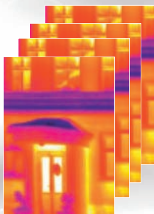
Термограммы 1-4
