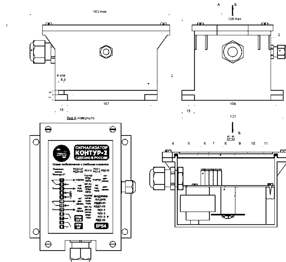
Рис. 1. Конструкция сигнализатора «Контур-2» (модификация «РСУ-3»).
