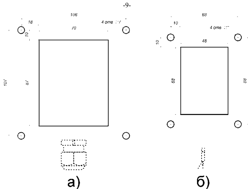
Рис. 6. Установочные отверстия для монтажа сигнализатора «Контур-2» (а) и детектора ППМ-02Пр (б).
