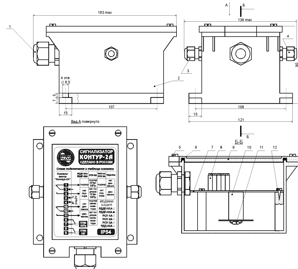
Рис. 1. Конструкция сигнализатора «Контур-2А» (модификация «РДДП-02А»).
