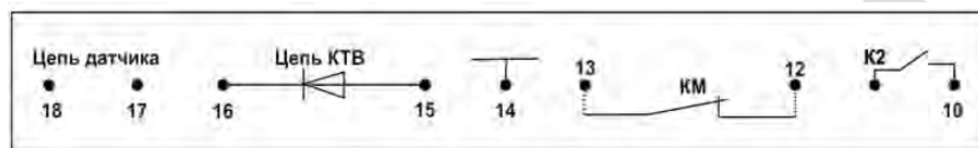
ЦЕПЬ ДАТЧИКА
