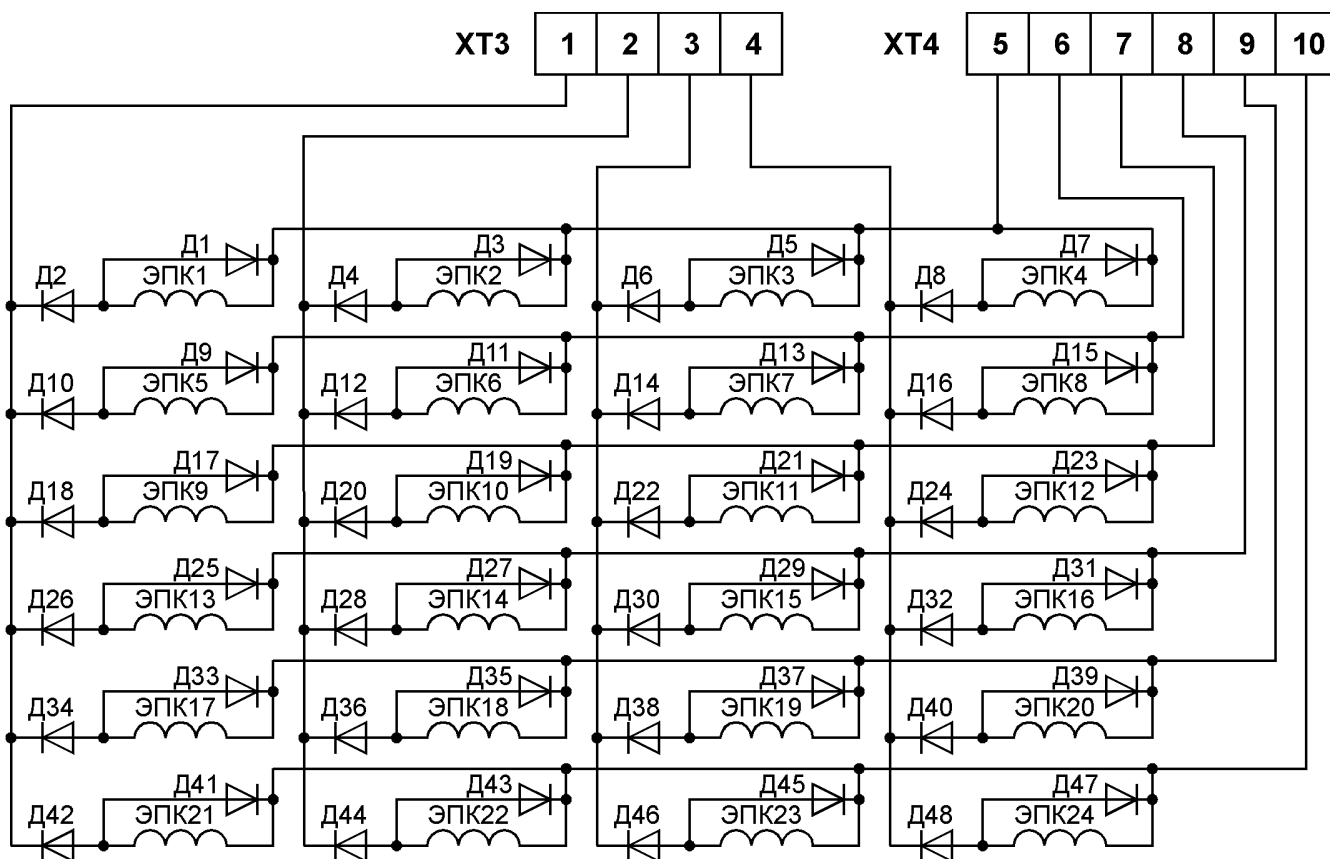
Рис. 3. Схема подключения ЭПК.
