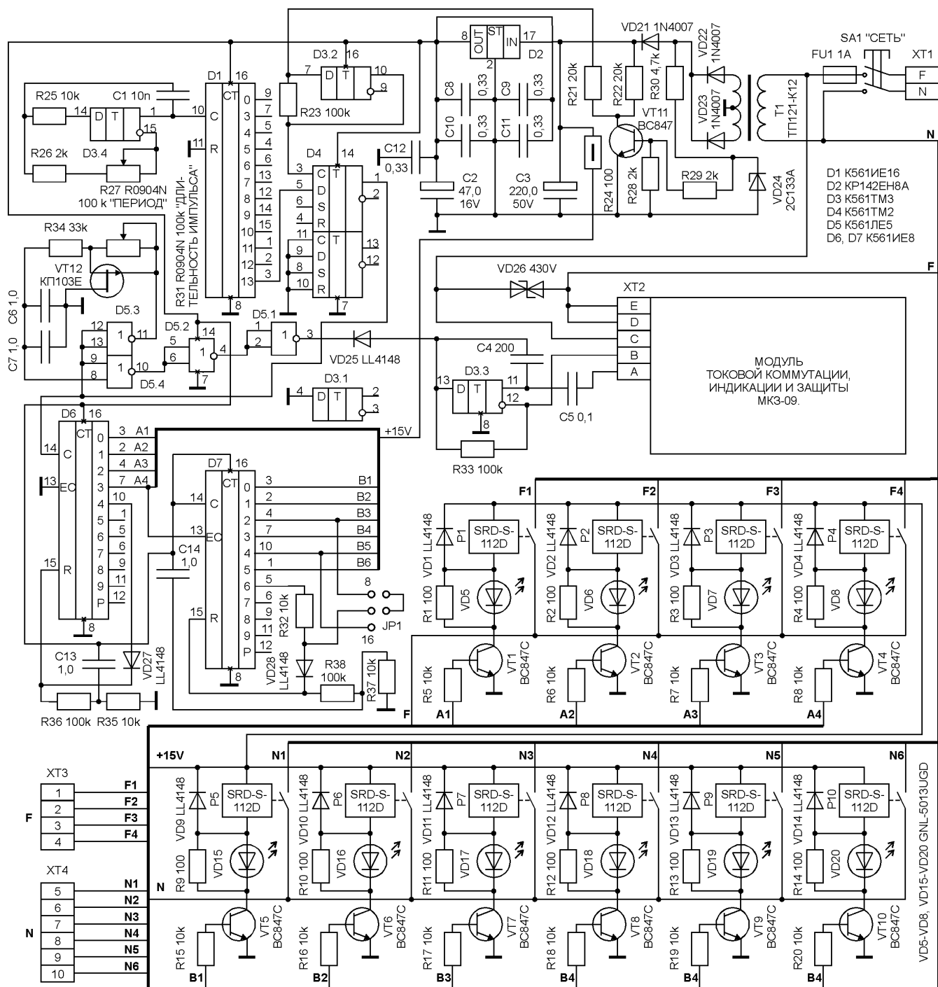
Рис. 2. Принципиальная электрическая схема блока А-03.
