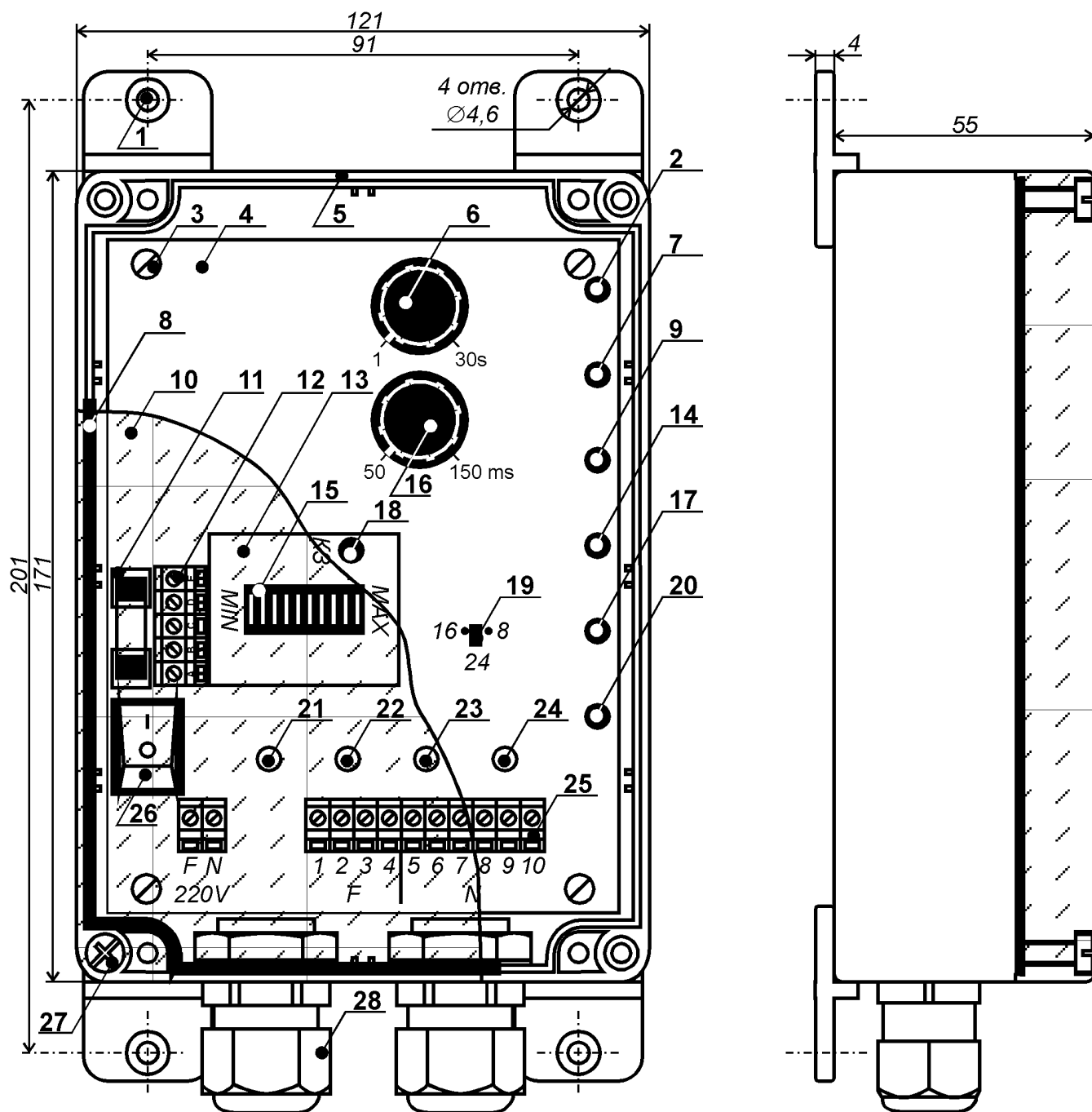
Рис. 1. Конструкция блока А-03.
