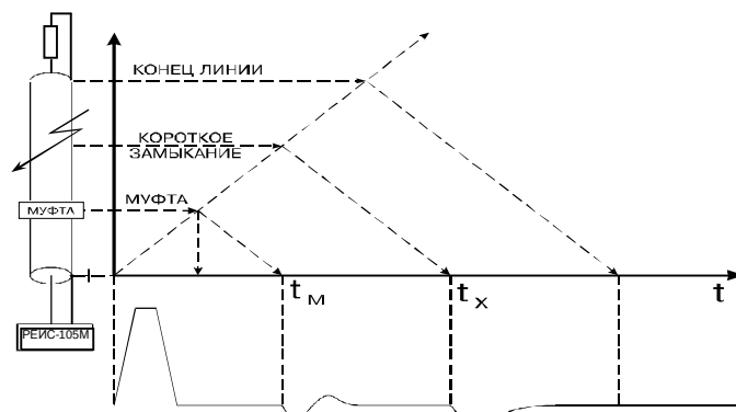
Рисунок 2 - Рефлектометрический метод определения места повреждения
