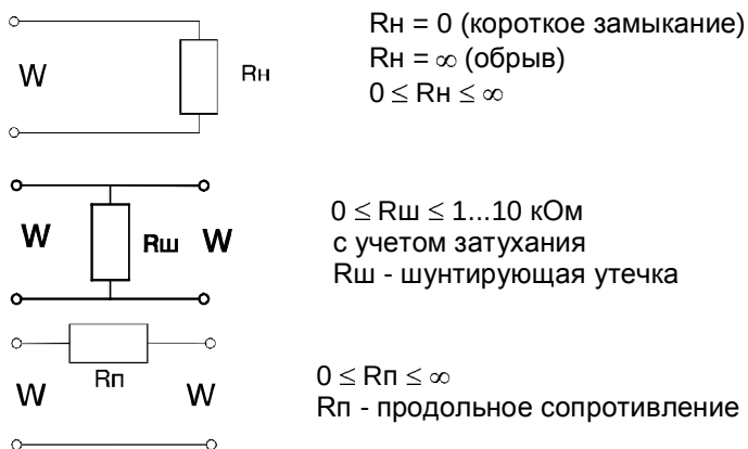
Рисунок 3 - Эквивалентные схемы повреждений
