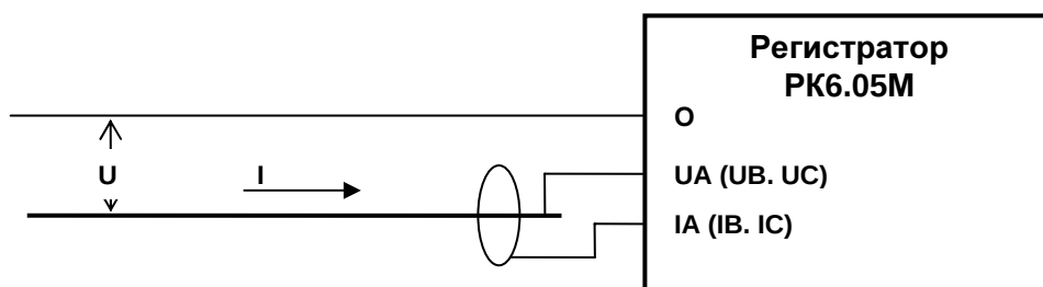
Рисунок 6 – Схемы подключения регистратора к однофазной электрической сети
