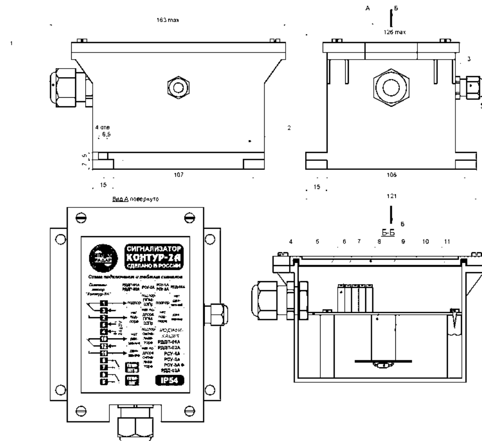
Рис. 1. Конструкция сигнализатора «Контур-2А» (модификация «РСУ-3А»).
