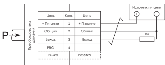
Схема подключения преобразователей общепромышленного исполнения
