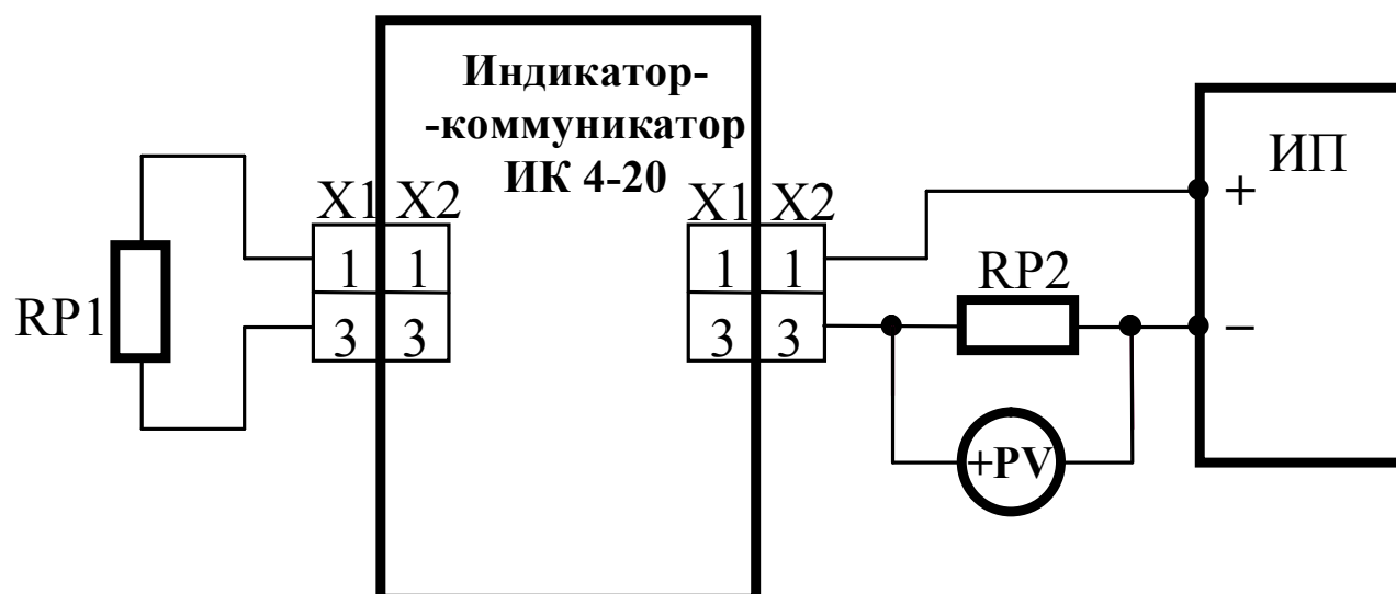
Рисунок Б.1 Схема подключения ИК 4-20 к контрольно-измерительному оборудованию при калибровке.
