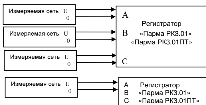
Рисунок 5а Подключение регистратора при измерении в однофазной сети
