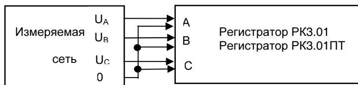
Рисунок 5б Подключение регистратора при трехфазном четырех проводном соединении(схема .Звезда.)
