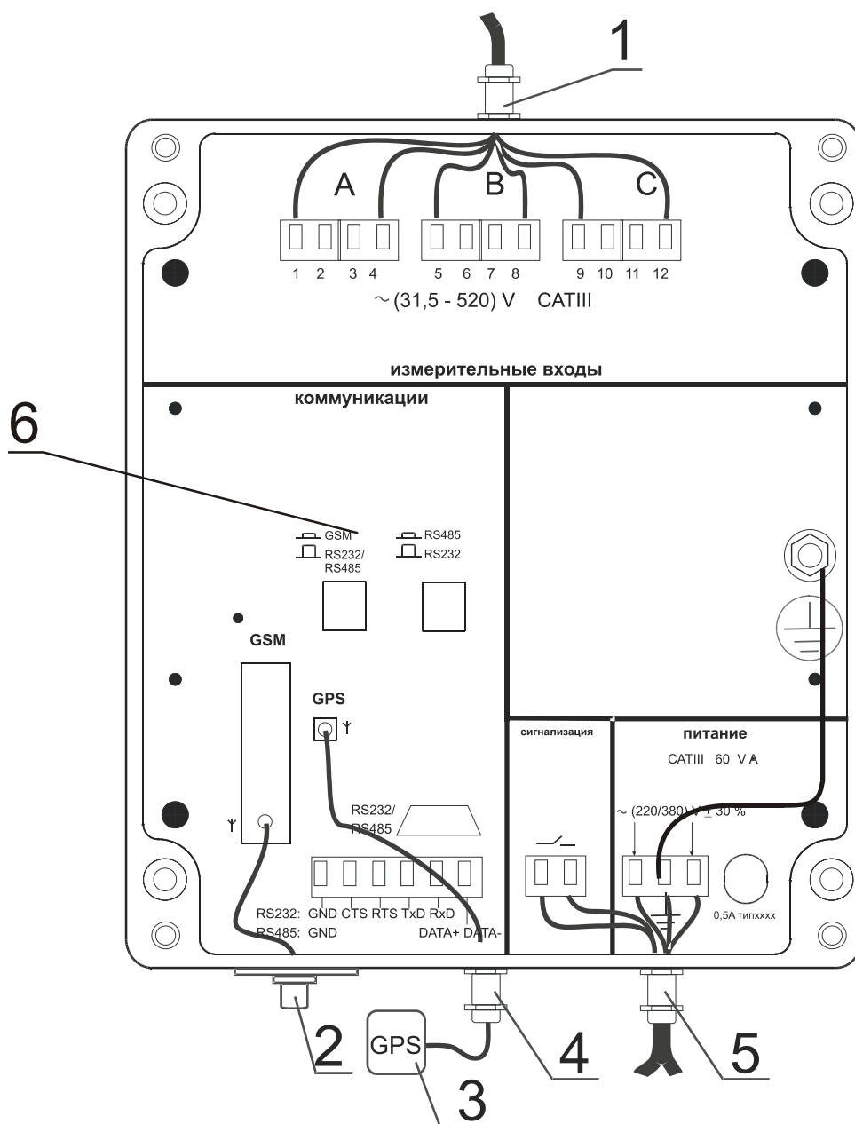
Рисунок А.12 Вариант исполнения и схема подключения регистратора показателей качества электрической энергии «Парма РК3.02-11»
