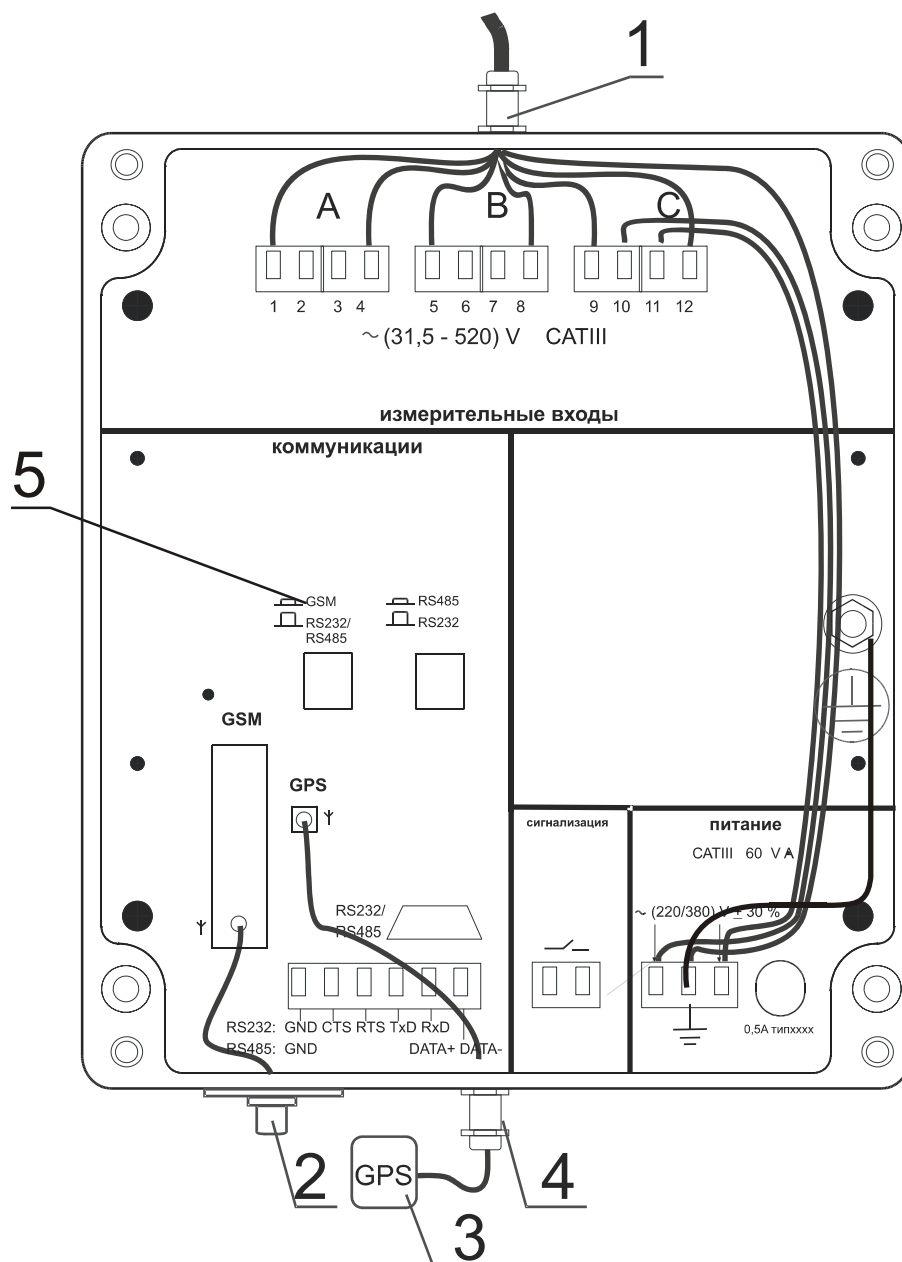
Рисунок А.10 Вариант исполнения и схема подключения регистратора показателей качества электрической энергии «Парма РК3.02-09»
