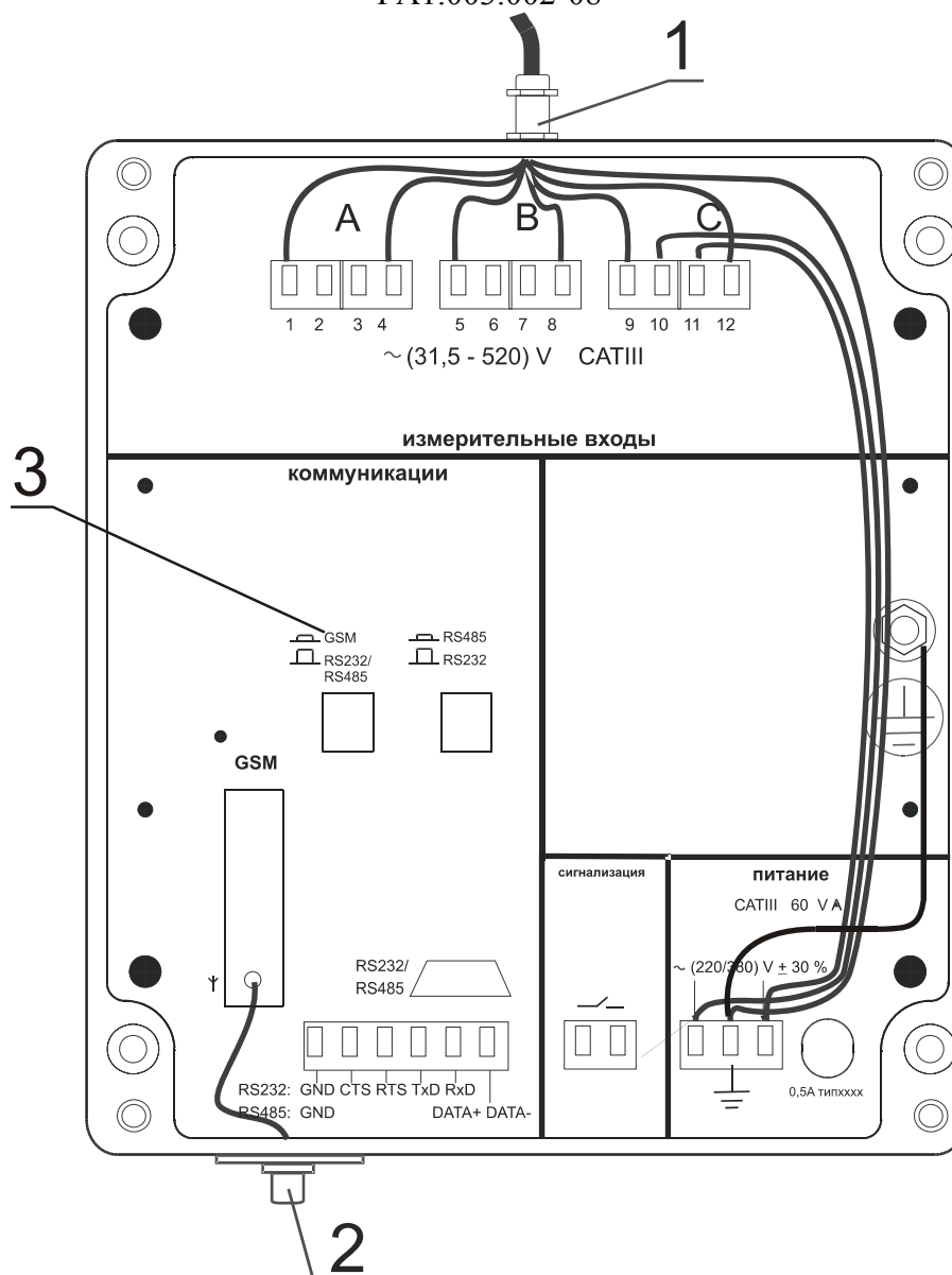
Рисунок А.9 Вариант исполнения и схема подключения регистратора показателей качества электрической энергии «Парма РК3.02-08»
