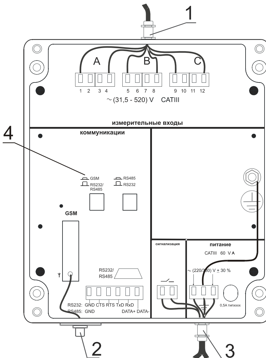
Рисунок А.11 Вариант исполнения и схема подключения регистратора показателей качества электрической энергии «Парма РК3.02-10»
