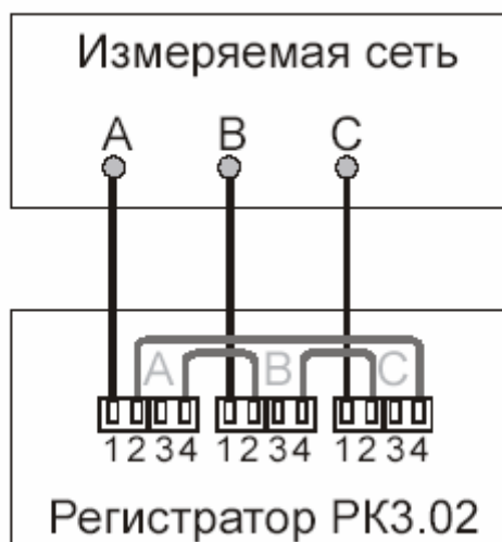
Рисунок 6 Схема подключения измерительных входов регистратора при 3-х проводной схеме подключения
