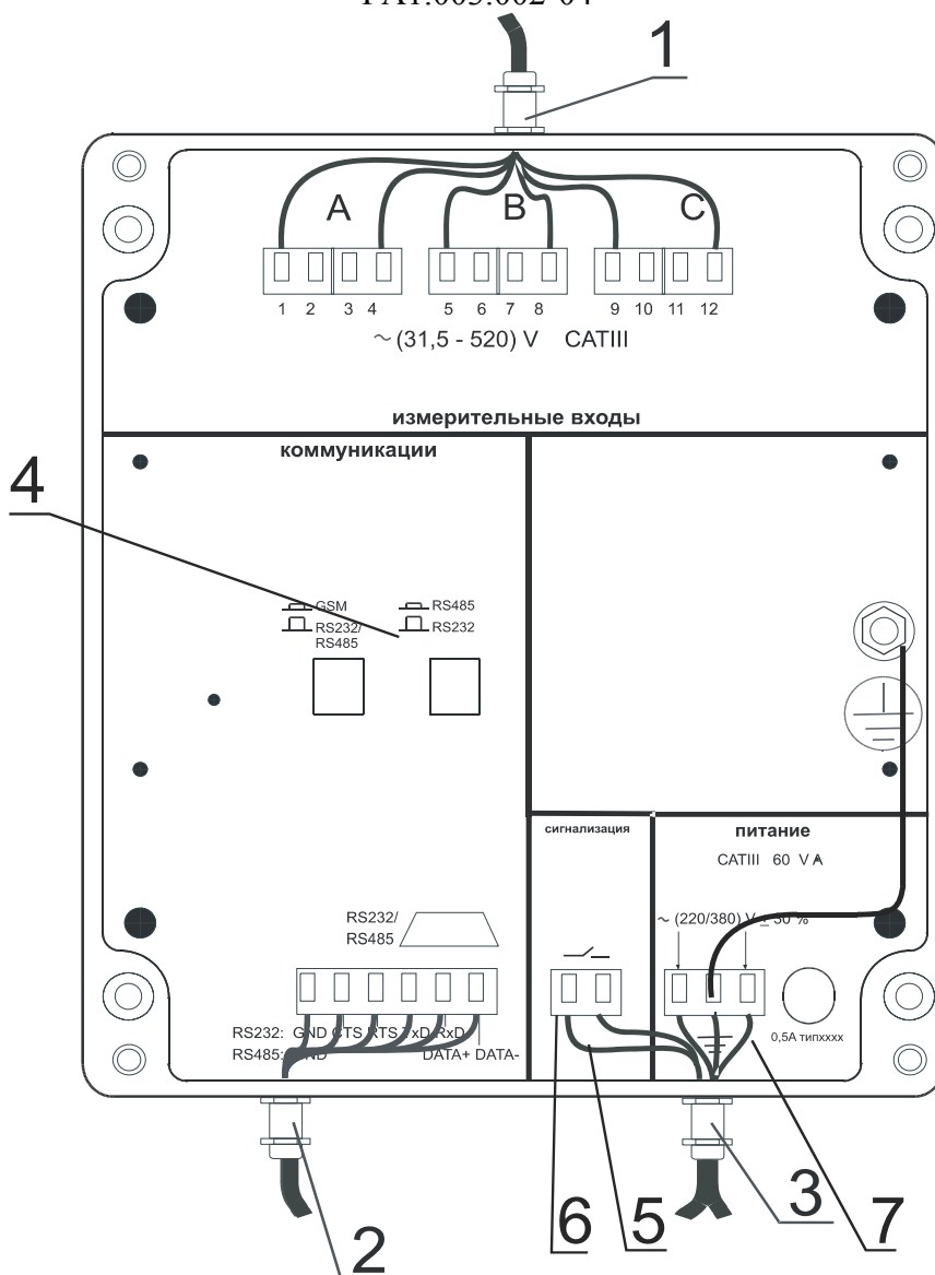
Рисунок А.5 Вариант исполнения и схема подключения регистратора показателей качества электрической энергии «Парма РК3.02-04»
