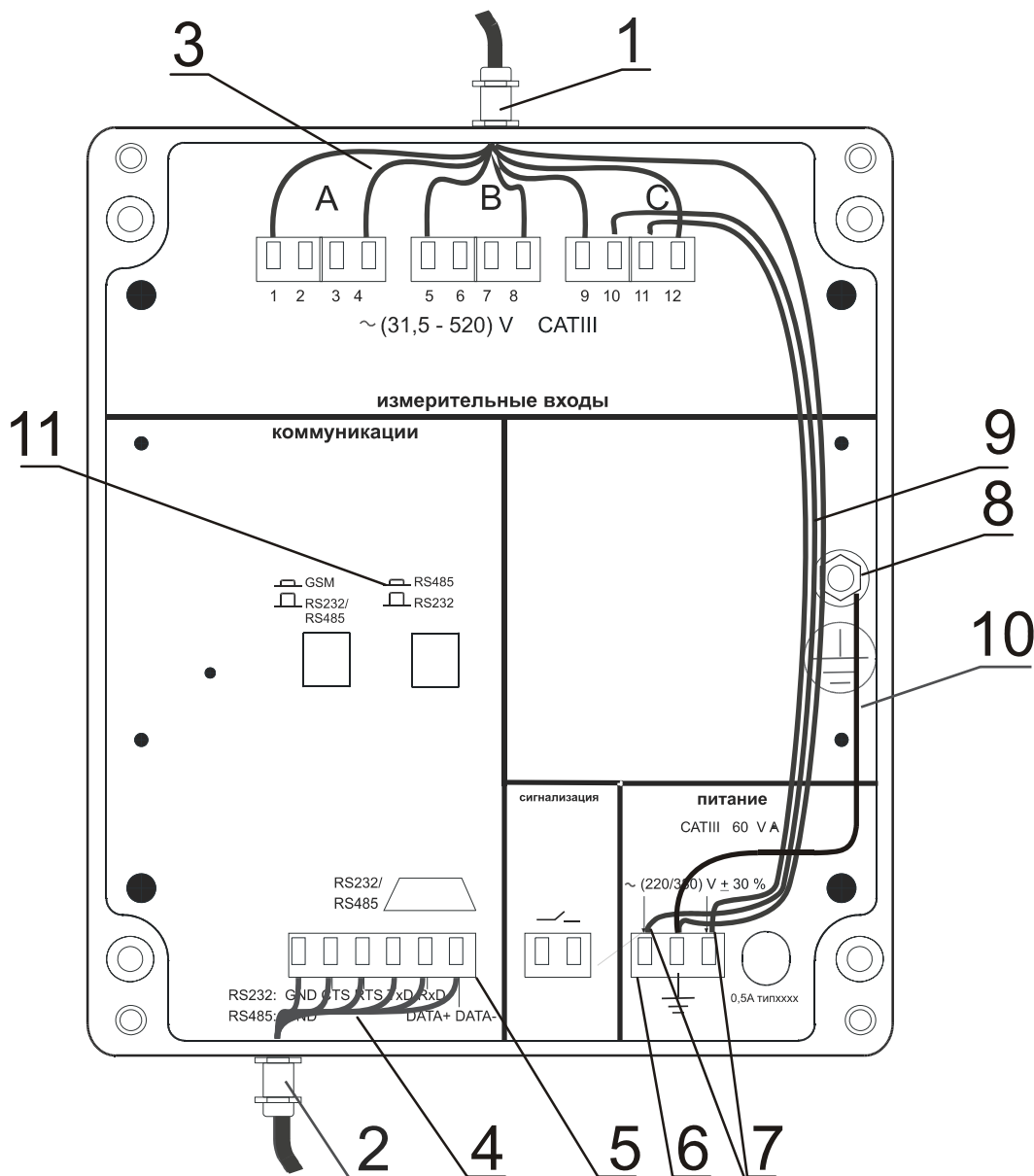
Рисунок А.1 Вариант исполнения и схема подключения регистратора показателей качества электрической энергии «Парма РК3.02»
