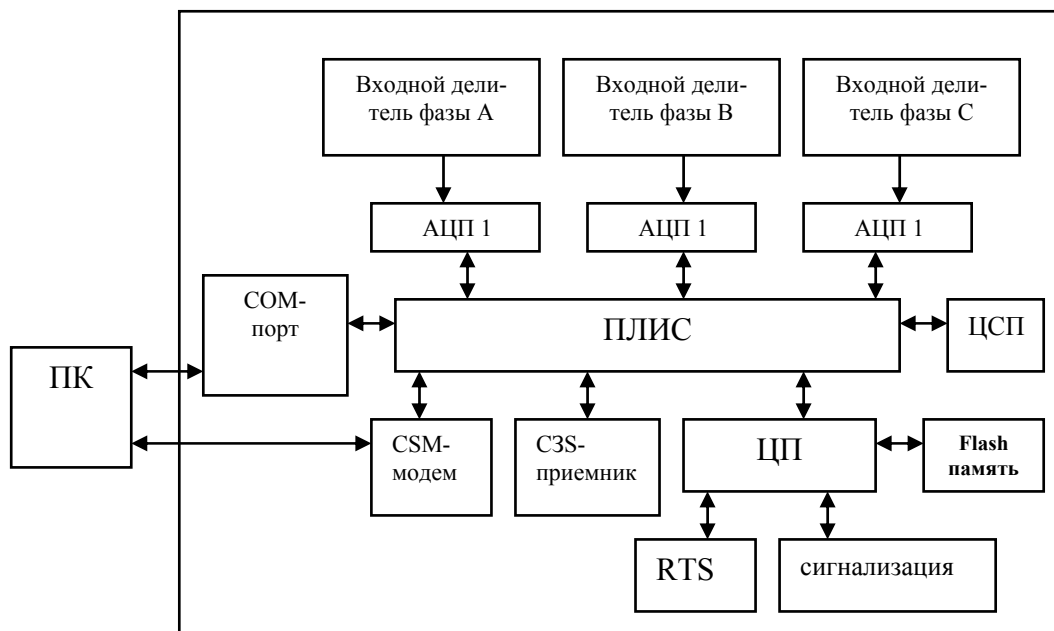
Рисунок 2 Структурная схема регистратора
