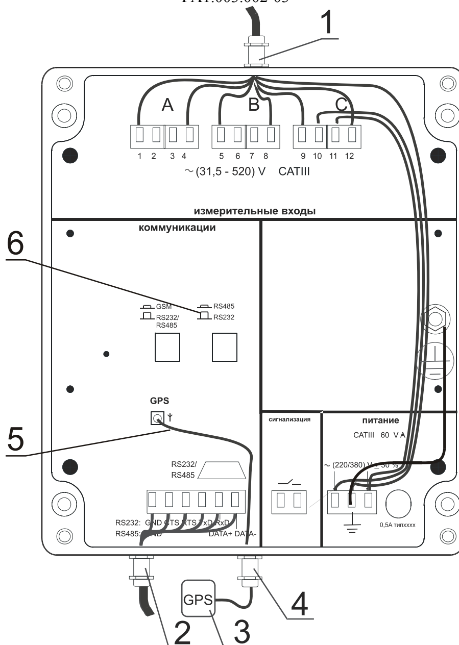
Рисунок А.4 Вариант исполнения и схема подключения регистратора показателей качества электрической энергии «Парма РК3.02-03»
