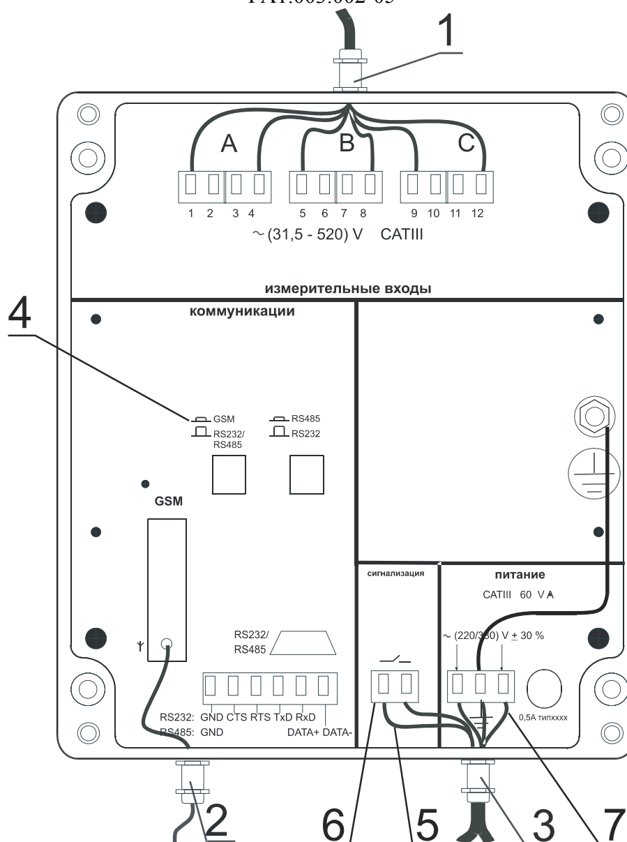
Рисунок А.6 Вариант исполнения и схема подключения регистратора показателей качества электрической энергии «Парма РК3.02-05»
