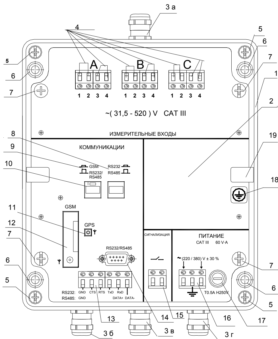
Рисунок 2 Внешний вид основания корпуса регистратора
