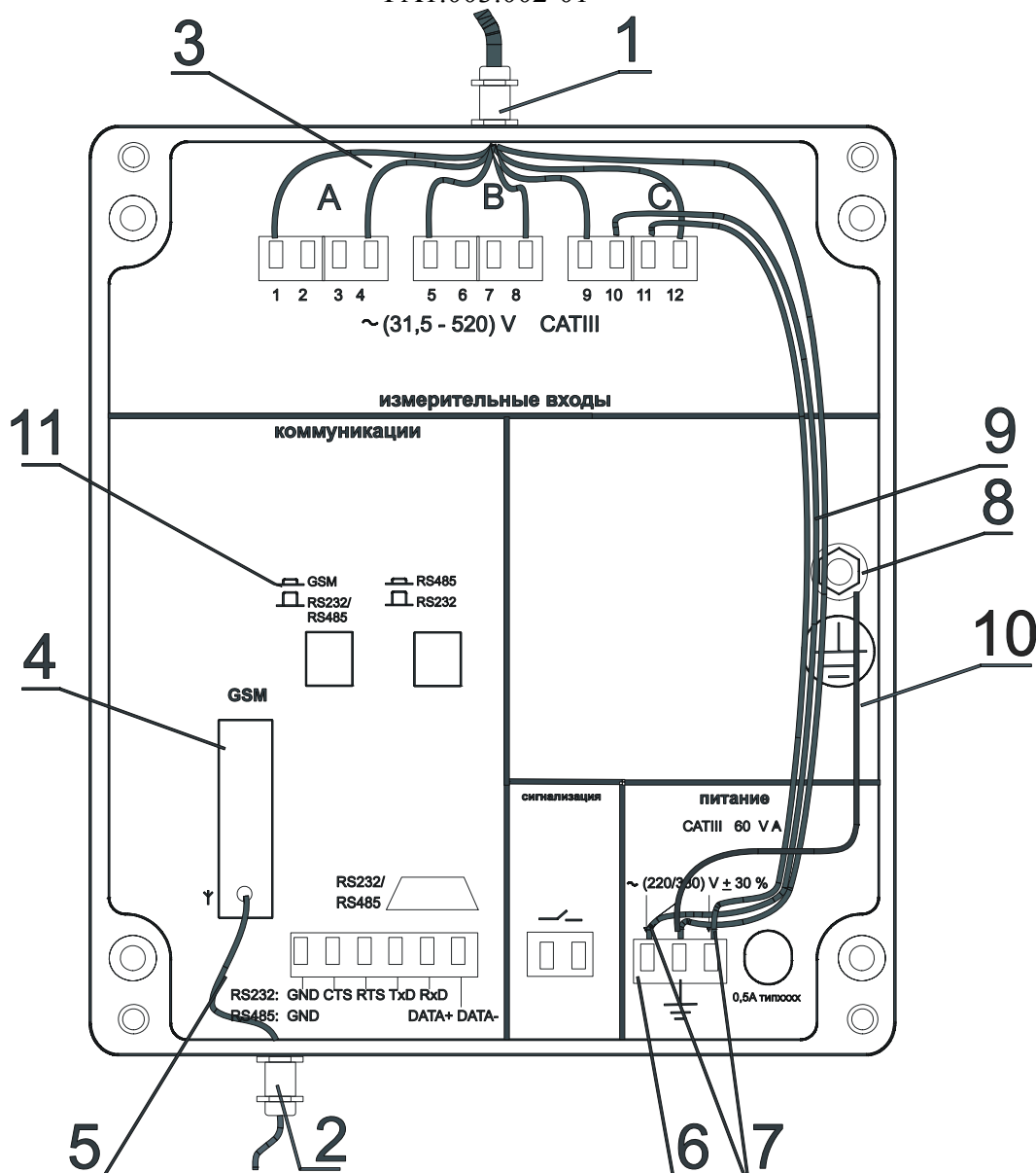
Рисунок А.2 Вариант исполнения и схема подключения регистратора показателей качества электрической энергии «Парма РК3.02-01»
