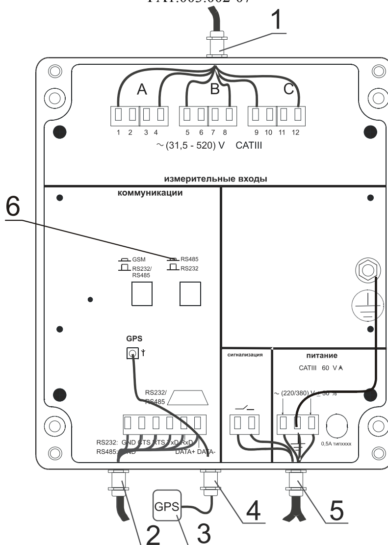
Рисунок А.8 Вариант исполнения и схема подключения регистратора показателей качества электрической энергии «Парма РК3.02-07»
