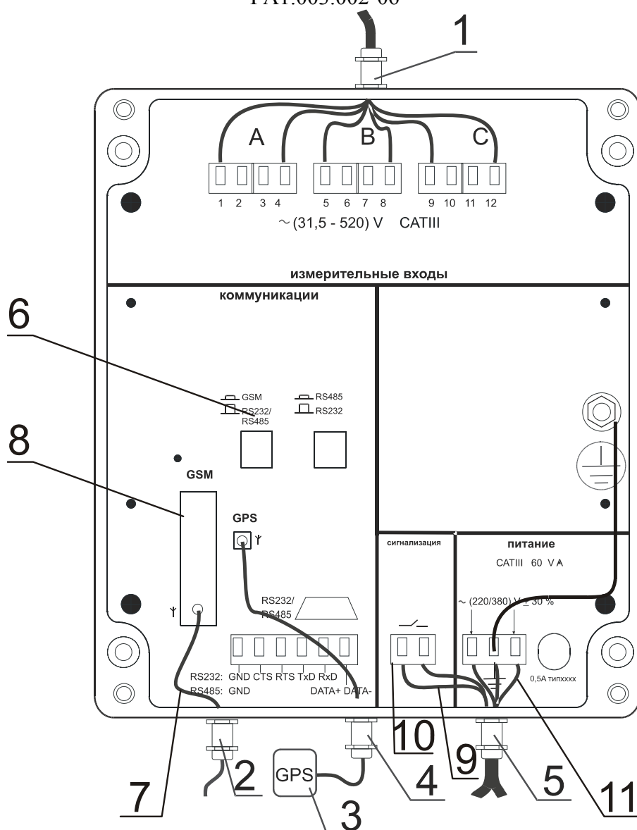
Рисунок А.7 Вариант исполнения и схема подключения регистратора показателей качества электрической энергии «Парма РК3.02-06»
