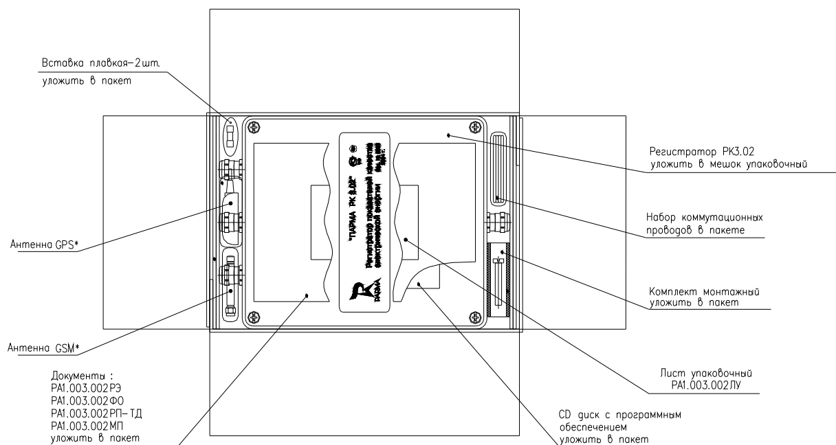
Рисунок 3 – Схема упаковки регистратора
