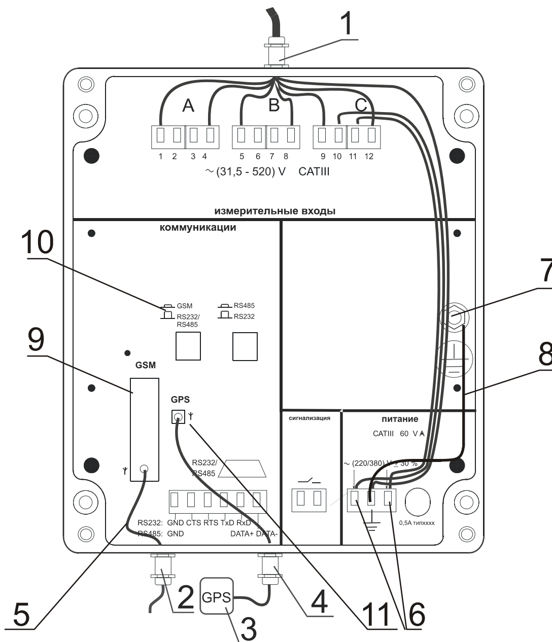
Рисунок А.3 Вариант исполнения и схема подключения регистратора показателей качества электрической энергии «Парма РК3.02-02»
