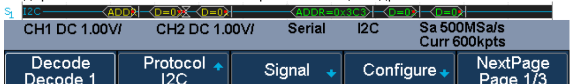
Рис. 12-4 Пример результата декодирования сигнала I2C
