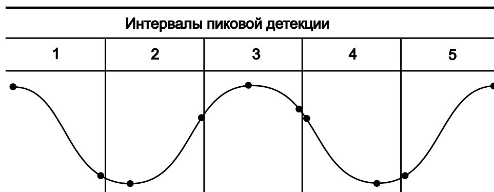
Рис. 10-5 Принцип формирования выборок пикового детектора
