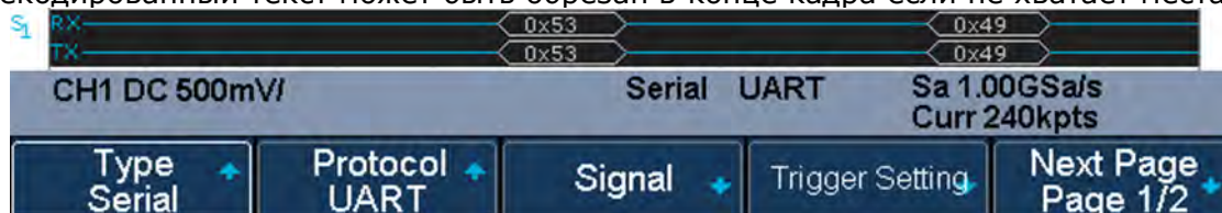
Рис. 12-14 Пример результата декодирования сигнала UART/RS232
