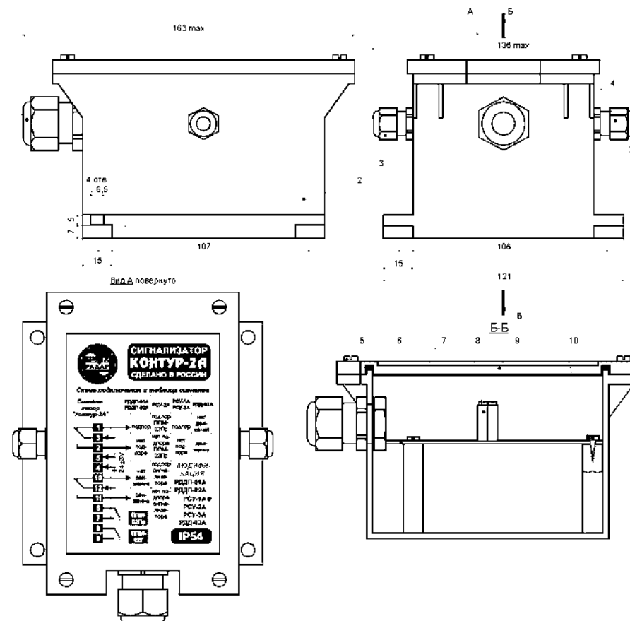
Рис. 4. Конструкция сигнализатора «Контур-2А» (модификация «PCY-1А»).
