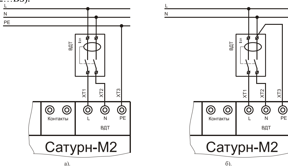
Рисунок В6 – Схемы подключения устройства «Сатурн-М2» при проверке ВДТ
