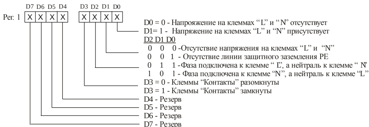
Рисунок 6 – Регистр состояния 1
