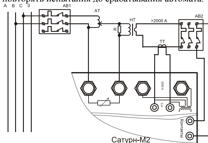
Рисунок В5 – Схема проверки автоматических выключателей синусоидальным током с помощью устройства «Сатурн-М3»
