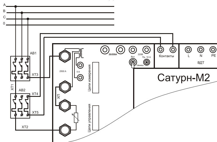
Рисунок В1 – Схема проверки автоматических выключателей с номинальными токами до 200 А с помощью устройства «Сатурн-М2»
