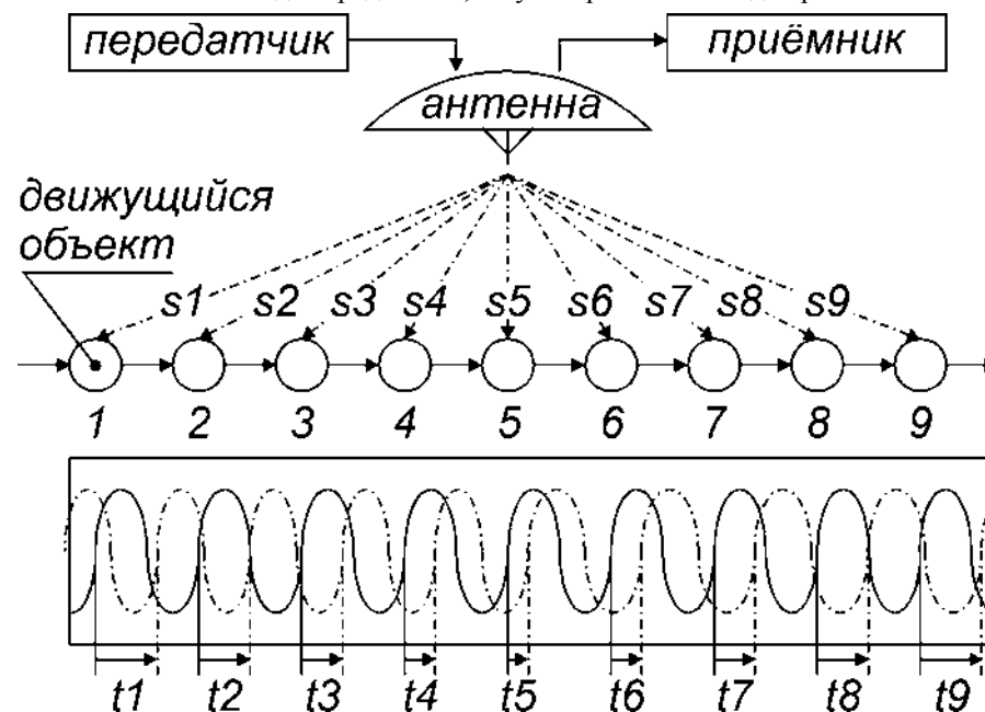
Рис. 3. Эффект Допплера.
