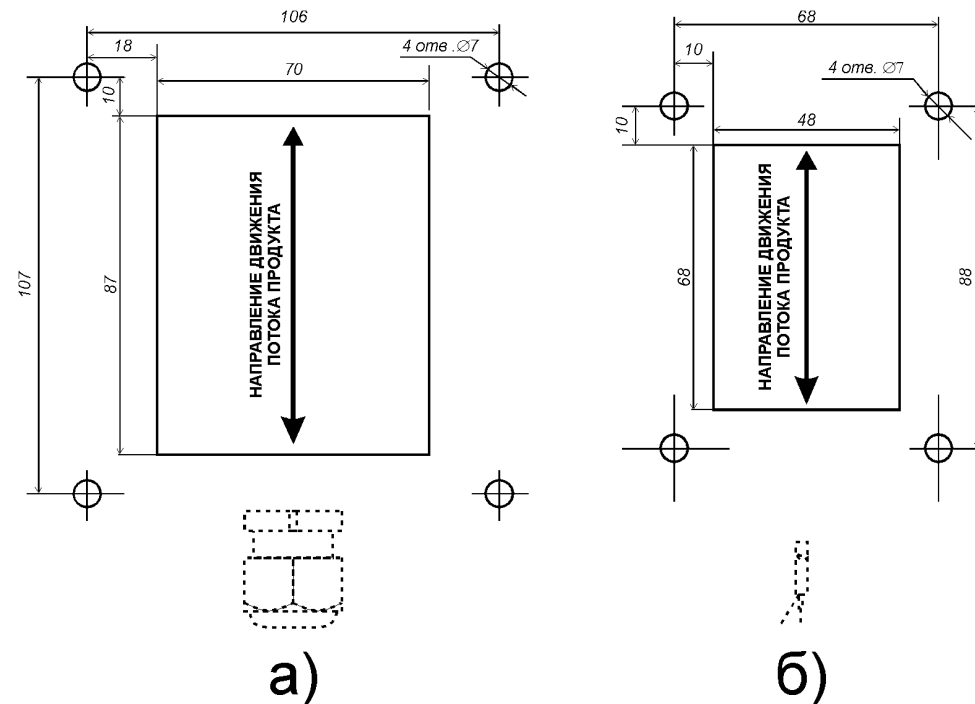
Рис. 7. Установочные отверстия для монтажа сигнализатора «Контур-2А» (а) и детектора ППМ-02Пр (б).
