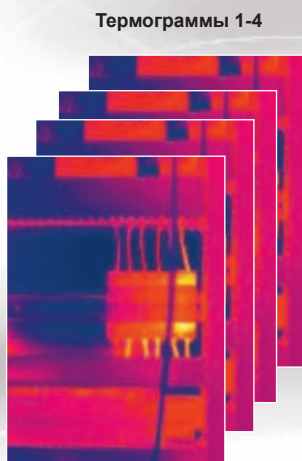
Термограммы 1-4
