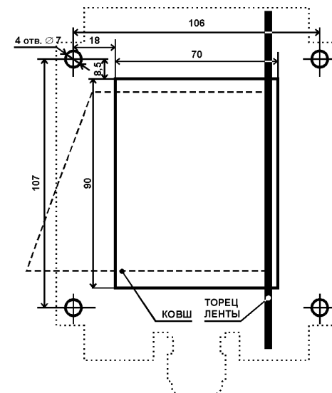
Рис. 6Б. Монтаж ДС-3А на норию с пластиковыми ковшами.
