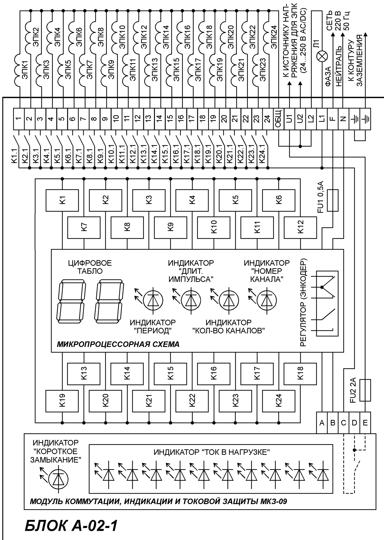
Рис. 2. Схема подключения и органы управления блока А-02-1.
