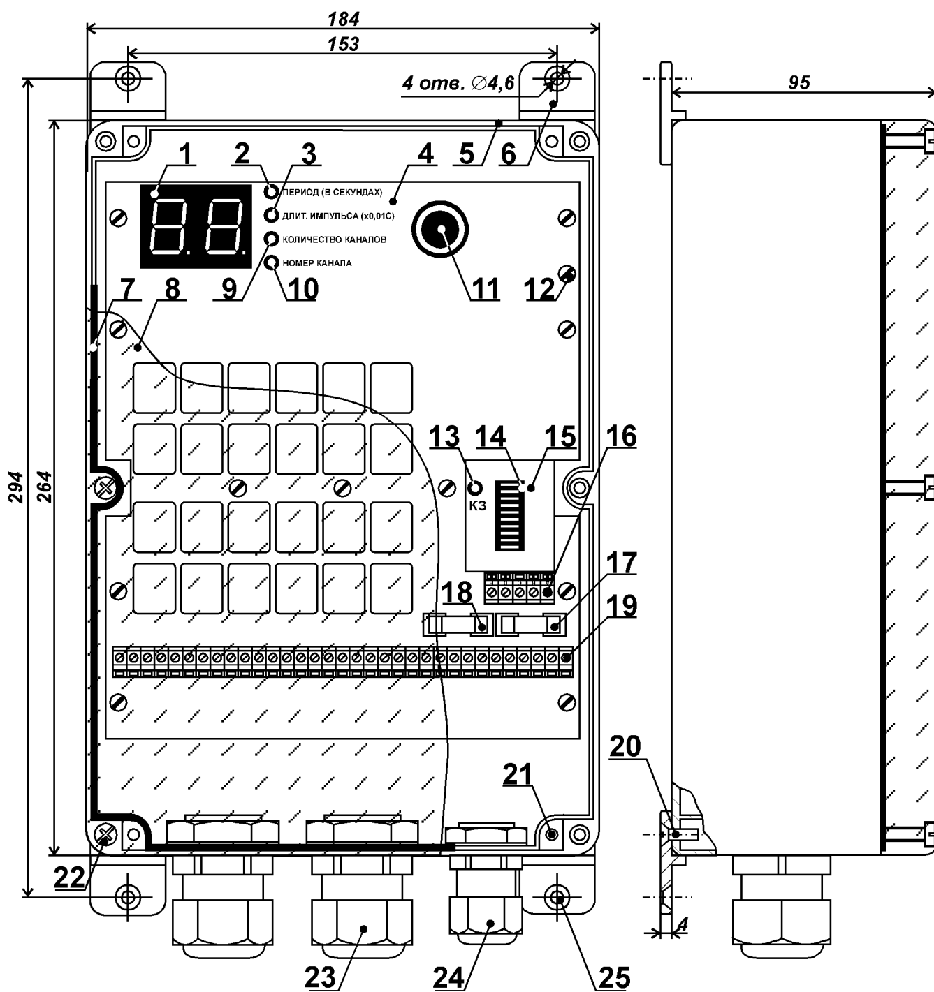
Рис. 1. Конструкция блока А-02-1.
