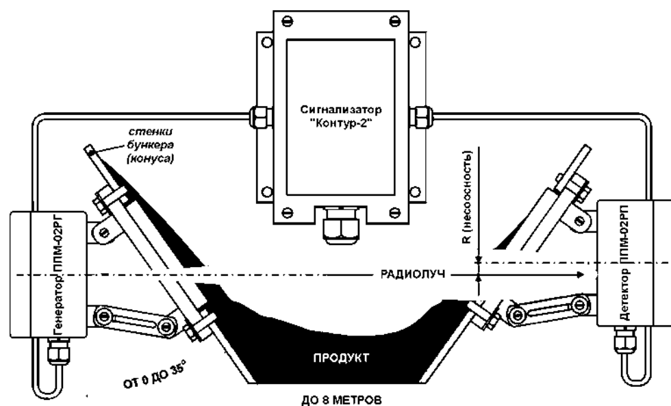
Рис. 1. Принцип действия датчика РСУ-1Р.
