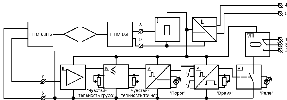
Рис. 4. Структурная схема датчика РСУ-1А.
