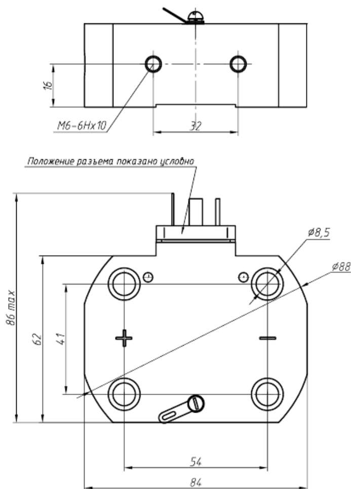
Рисунок Б.9 — Габаритный чертёж преобразователей избыточного давления, разрежения, давления-разрежения исполнения ВТ2 с кодом присоединительного размера 2 (по таблице А.8) и кодом конструктивного исполнения К20, К34 (по таблице А.14)
