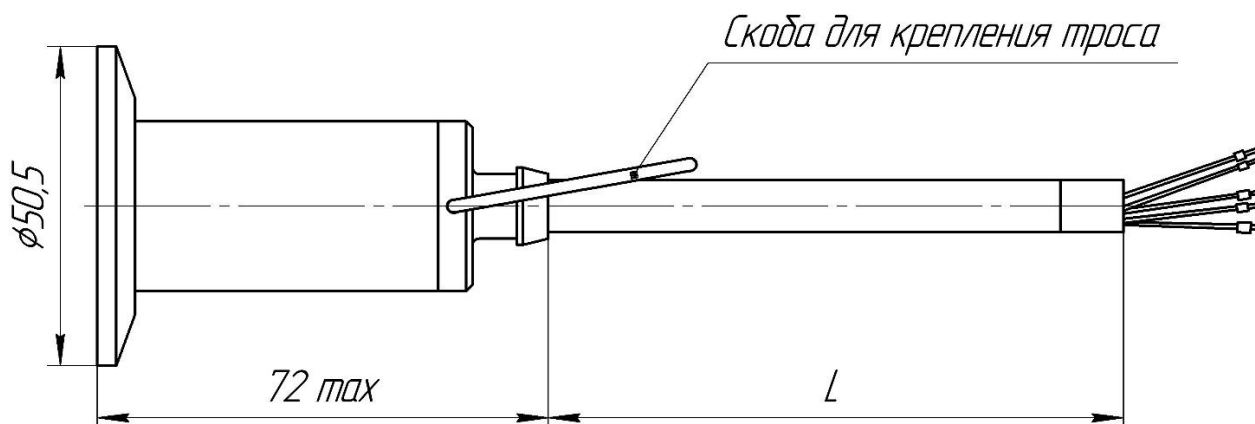
Рисунок Б.14 — Габаритный чертеж преобразователей гидростатического давления с кодом D20 по таблице А.1 , кодом присоединительного размера 5 по таблице А.8 и кодом конструктивного исполнения K05 по таблице А.14.
