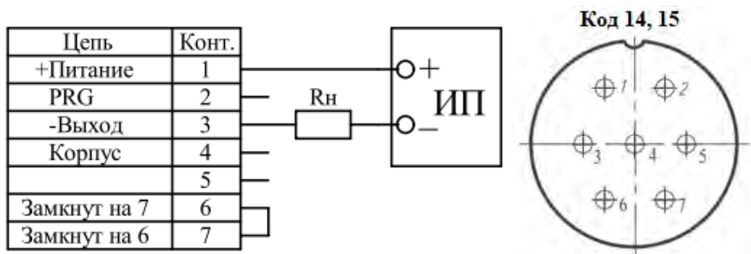
Рисунок В.3 — Соответствие цепей выводам разъёма преобразователей с кодами исполнений 14 и 15 по таблице А.10
