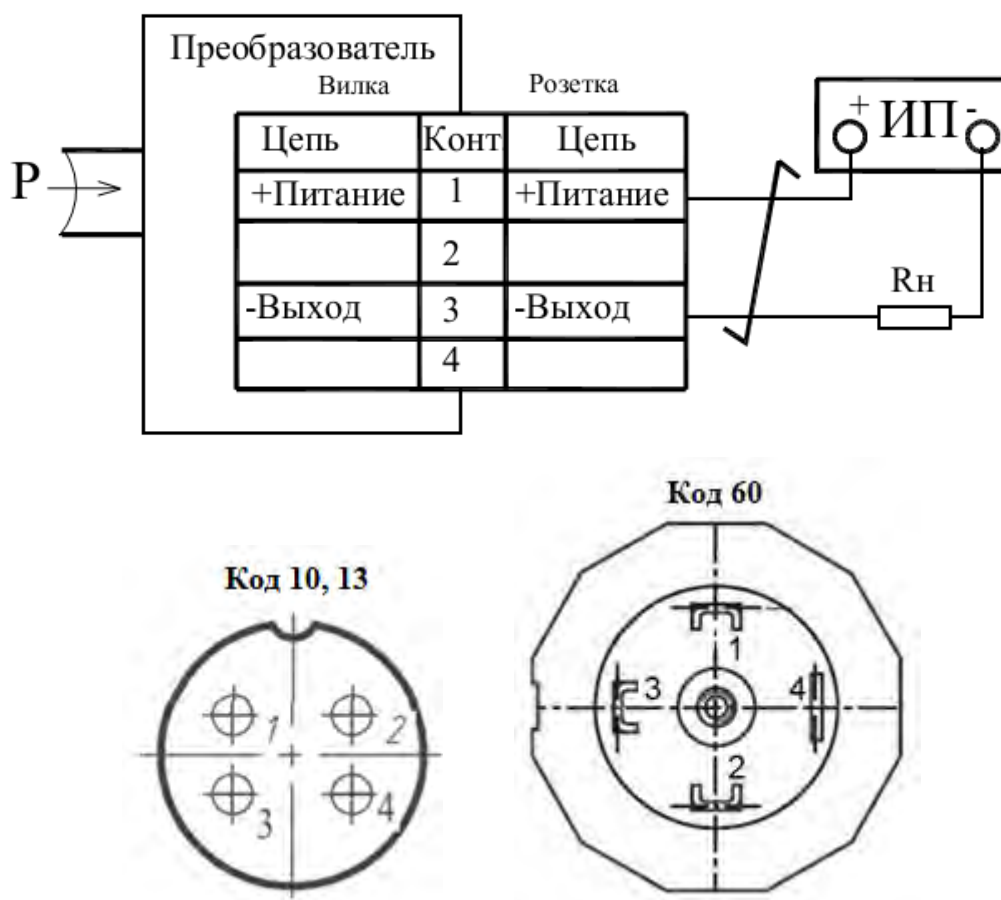
Рисунок В.1 — Схема подключения преобразователей общепромышленного исполнения с кодами 10, 13, 60 по таблице А.10
